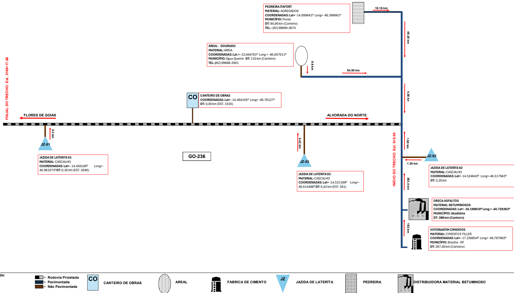
Figura 2 - Diagrama Linear de Obras com Localização das Fontes de Materiais.
