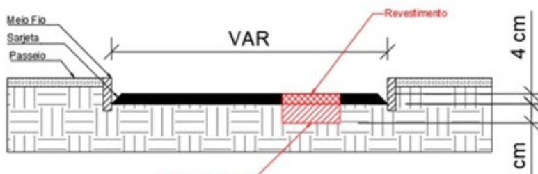
Figura 02 – Esquema de perfil transversal para reparo profundo.
