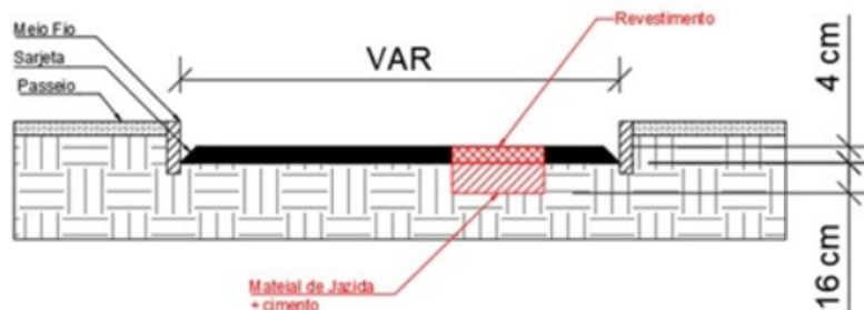
Figura 02 – Esquema de perfil transversal para reparo profundo.
