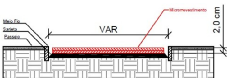
Figura 04 – Esquema de perfil transversal para Microrrevestimento.
