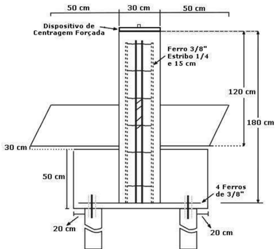
Figura 2 - Modelo de marco em formato de pilar de concreto - Fonte: Padronização de marcos geodésicos, 2008.
