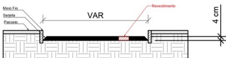
Figura 01 – Esquema de perfil transversal para reparo superficial.
