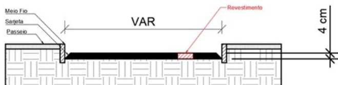
Figura 01 – Esquema de perfil transversal para reparo superficial.
