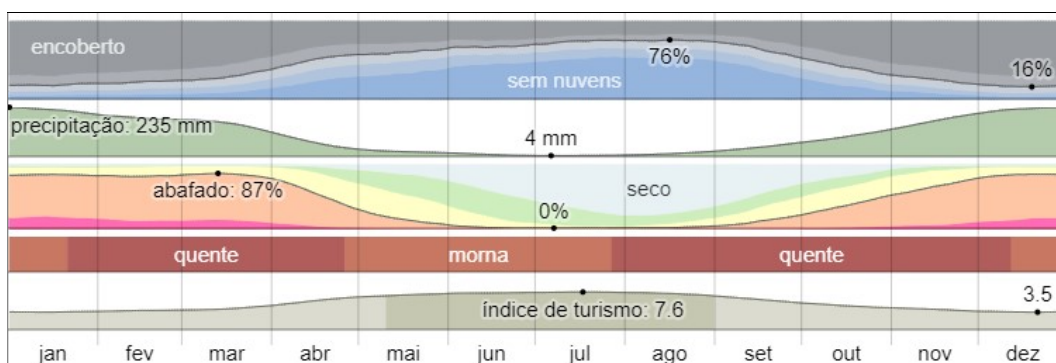
Figura 54 - Clima e condições meteorológicas médias em Caldas Novas ao longo do ano
