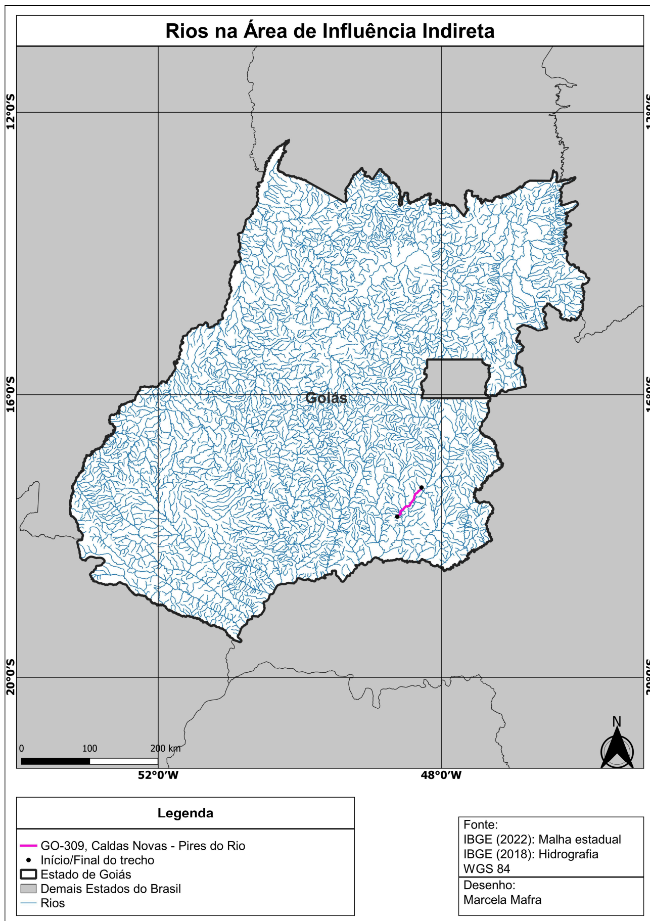
Figura 16 – Cursos d'água na AII
