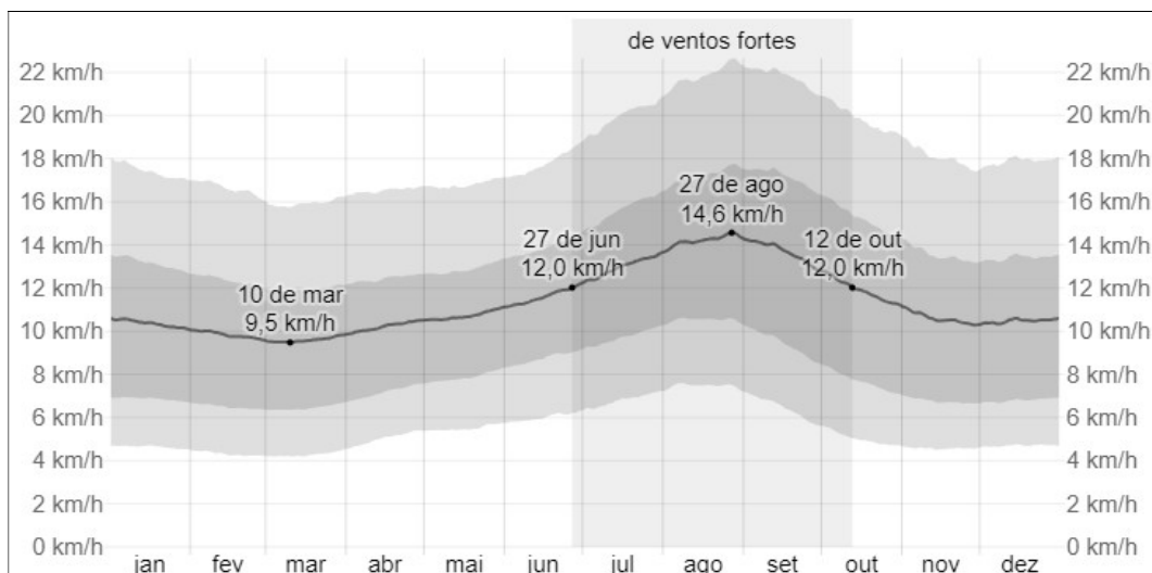
Figura 68 – Velocidade média do vento em Caldas Novas
