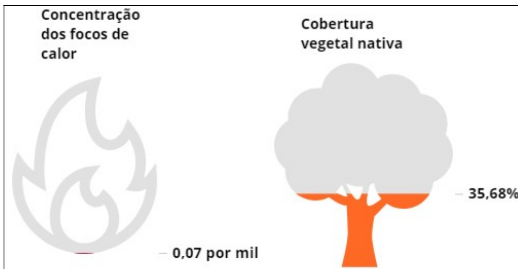
Figura 100 - Concentração dos focos de calor e cobertura vegetal por flora nativa no município de Caldas Novas/GO em 2017
