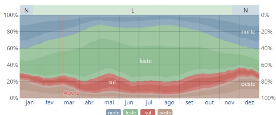
Figura 70 – Velocidade média do vento em Caldas Novas
