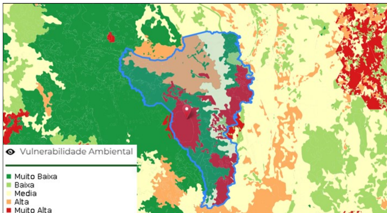
Figura 83 – Vulnerabilidade ambiental o município de Caldas Novas
