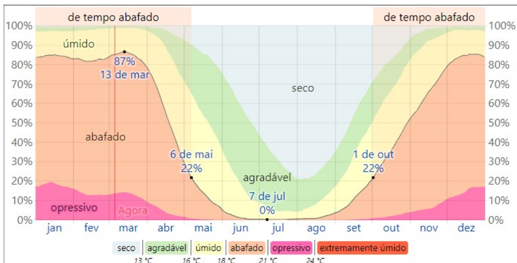
Figura 66 – Níveis de conforto em umidade em Caldas Novas
