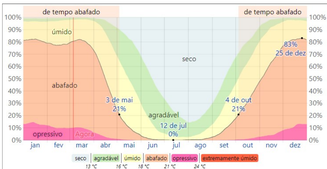
Figura 67 – Níveis de conforto em umidade em Pires do Rio
