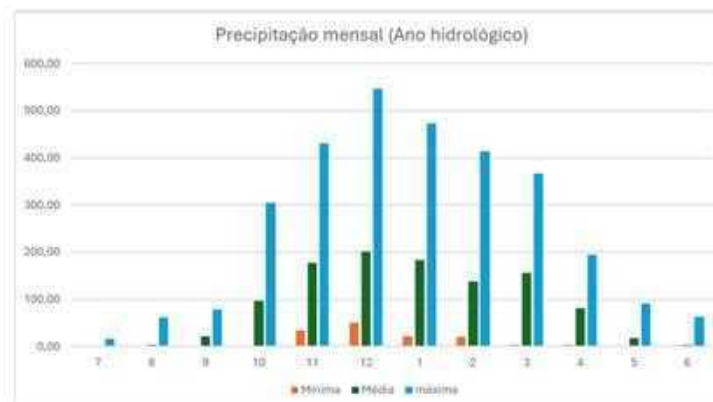
Figura 8 - precipitação na região do L5 - Ano Hidrológico
