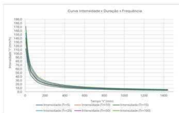
Figura 31 – Curva IDF na região do L3 – Posto Nova Roma
