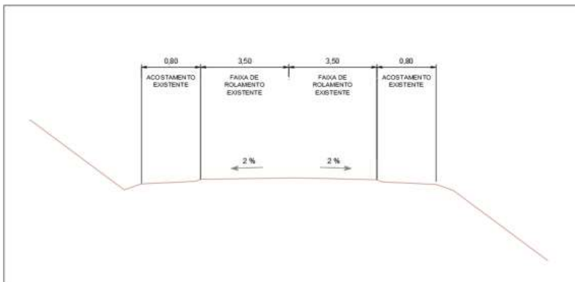
Figura 1 – Seção Tipo GO-217
