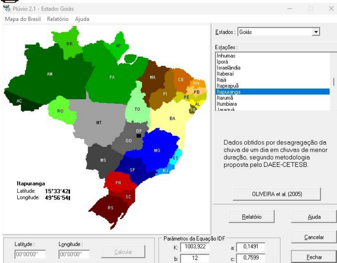
Figura 10. Parâmetros de equação de chuva do Município mais próximo a Faina - Itapuranga - GO
