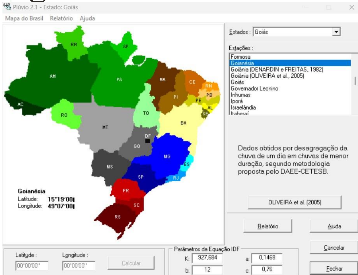
Figura 10. Parâmetros de equação de chuva do Município mais próximo a Itapaci - Goianésia - GO
