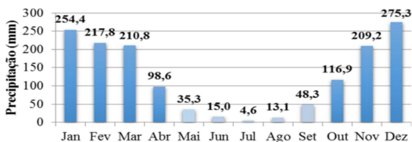
Figura 4. Gráfico de Precipitação Média Mensal no estado de Goiás.
