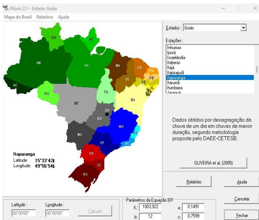
Figura 10. Parâmetros de equação de chuva do Município mais próximo a Morro Agudo de Goiás-GO. – Itapuranga-GO.
