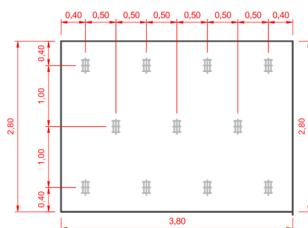
Figura 3 – Detalhe dos blocos de fundação – fundação proposta 2
