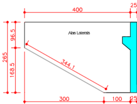
Figura 17 – Detalhe alas – Proposta 1
