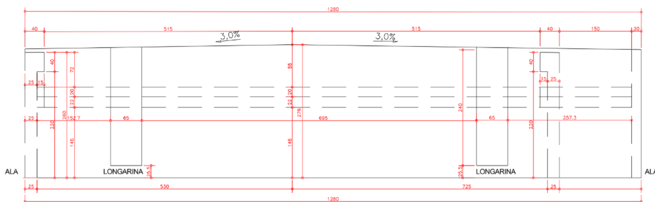
Figura 16 – Detalhe das travessas de apoio – Proposta 1
