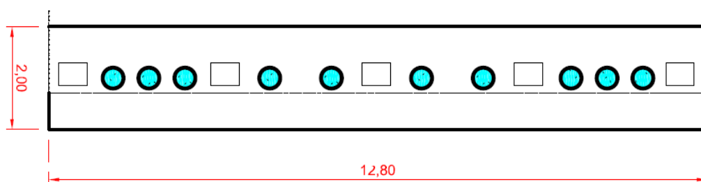
Figura 30 – Detalhe dos blocos de fundação – fundação proposta 1
