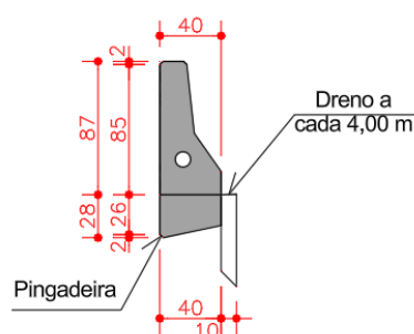
Figura 28 – Drenos e pingadeira – Proposta 1
