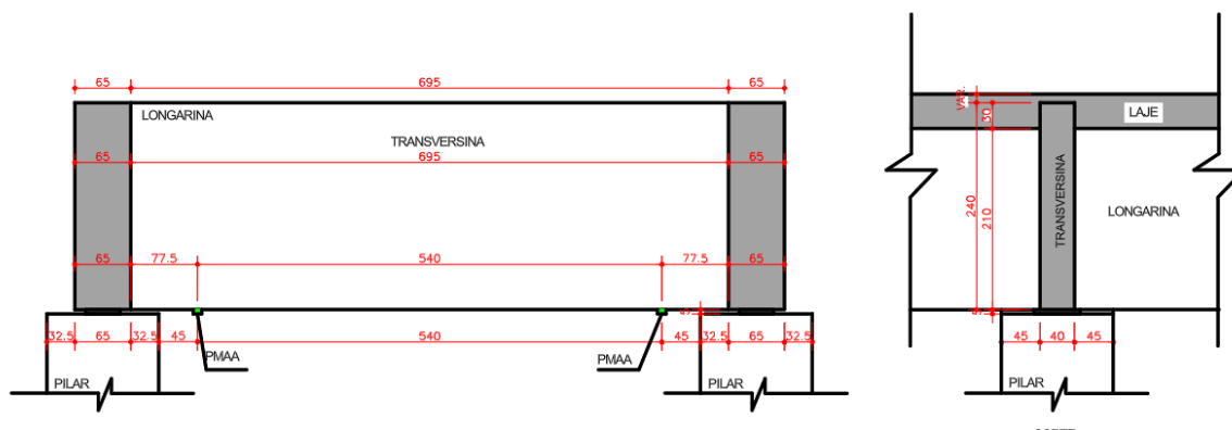
Figura 24 – Detalhe das transversinas de apoio – Proposta 2
