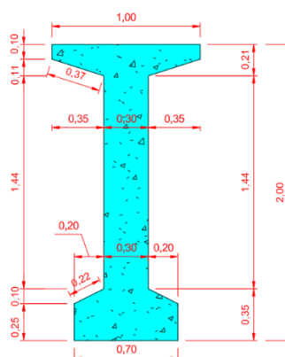
Figura 2 - Detalhes das longarinas – Proposta 1
