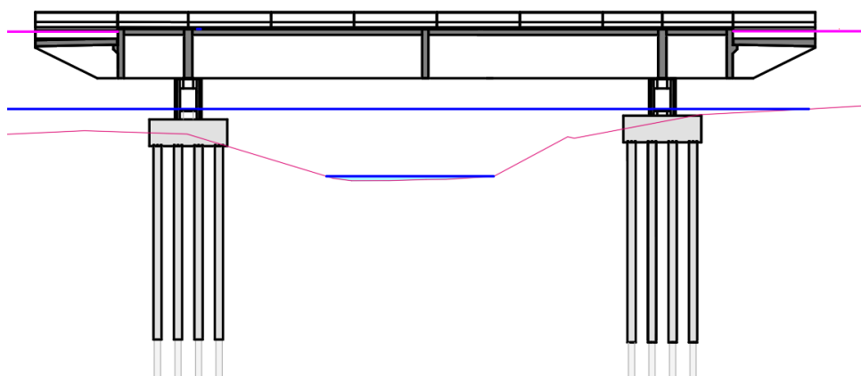
Figura 21 – Corte longitudinal – Proposta 2
