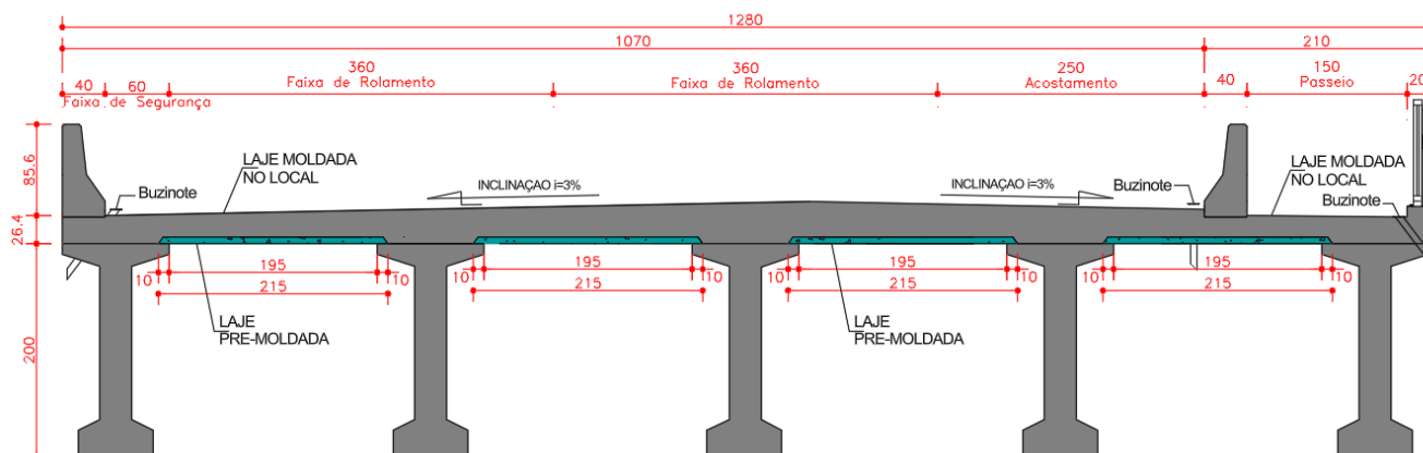
Figura 15 – Detalhe das lajes – Proposta 1
