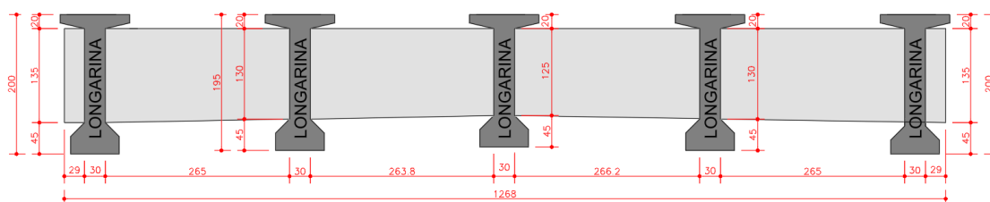
Figura 14 – Detalhe das transversinas vão – Proposta 1
