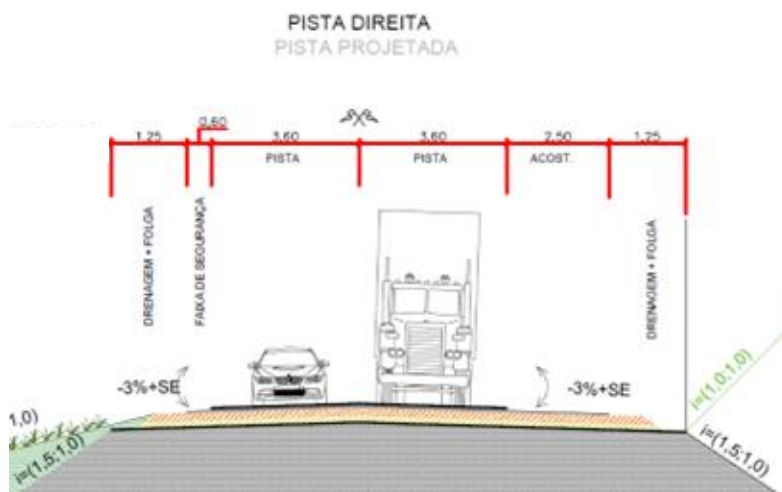
Figura 9 - Seção transversal típica
