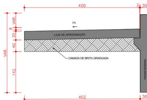
Figura 26 – Detalhe laje de aproximação – Proposta 2
