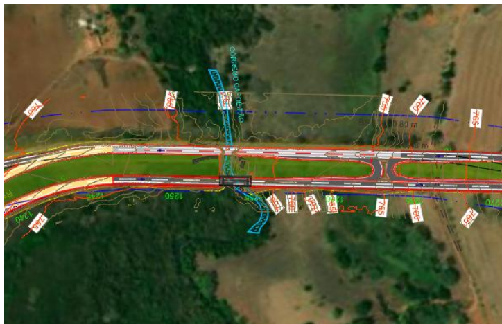
Figura 5 - Planta de localização
