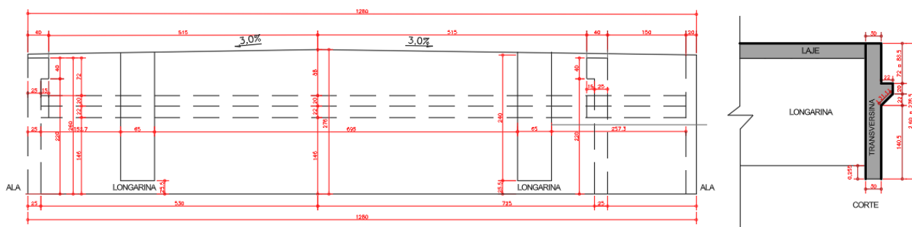
Figura 23 – Detalhe das transversinas de encontro – Proposta 2
