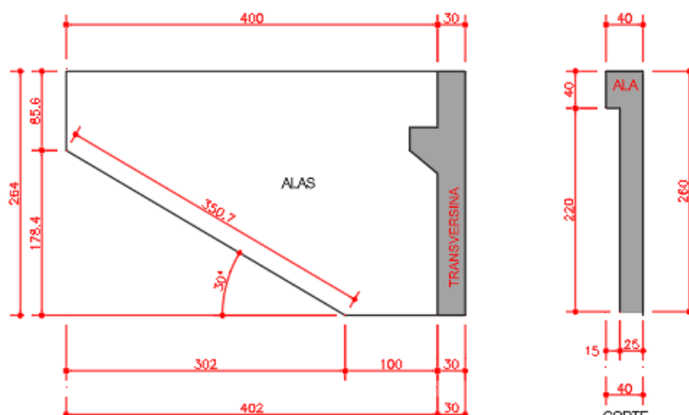
Figura 25 – Detalhe alas – Proposta 2
