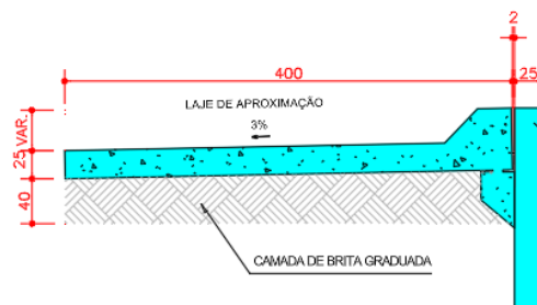
Figura 18 – Detalhe das lajes de aproximação – Proposta 1
