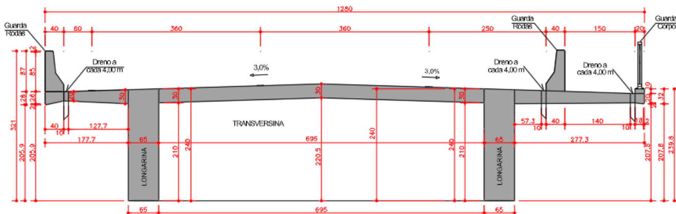
Figura 27 – Detalhe lajes – Proposta 2
