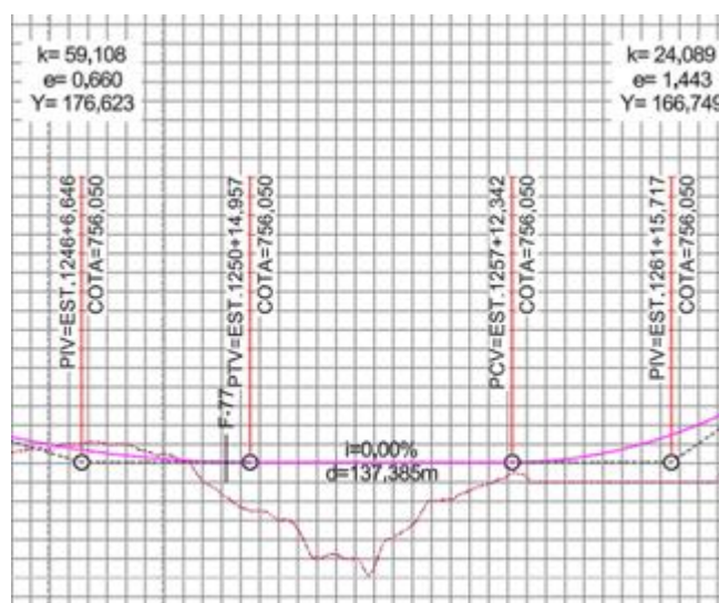
Figura 7 – Situação em Perfil
