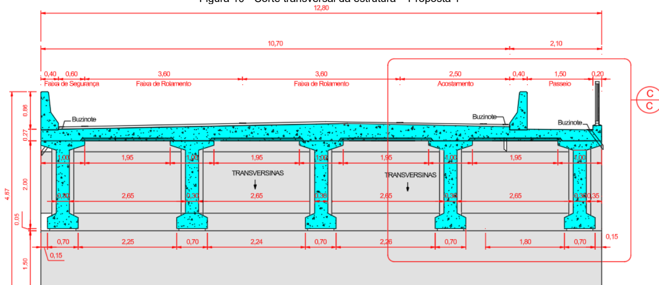
Figura 10 - Corte transversal da estrutura – Proposta 1
