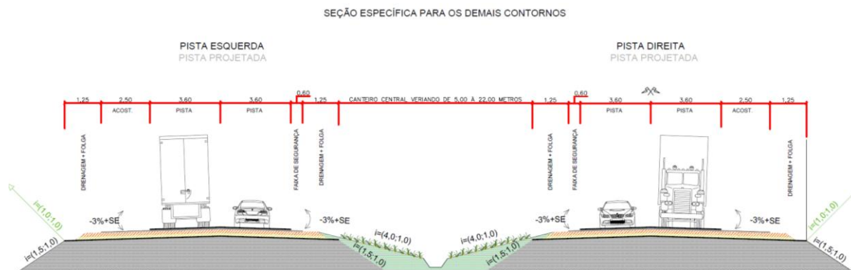
Figura 8 - Seção transversal típica
