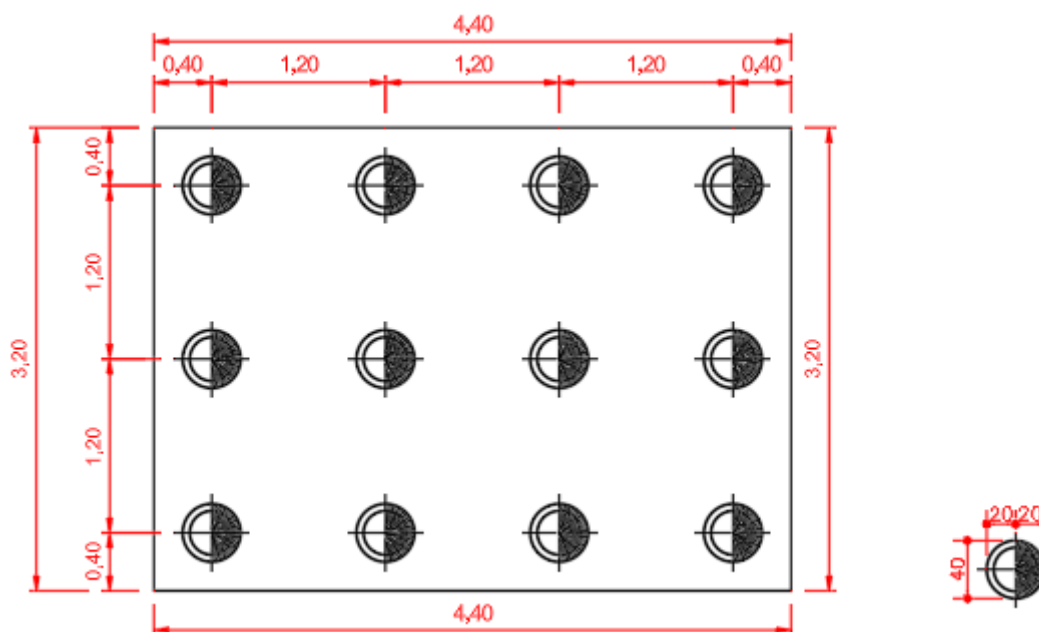
Figura 30 – Detalhe dos blocos de fundação – fundação proposta 1
