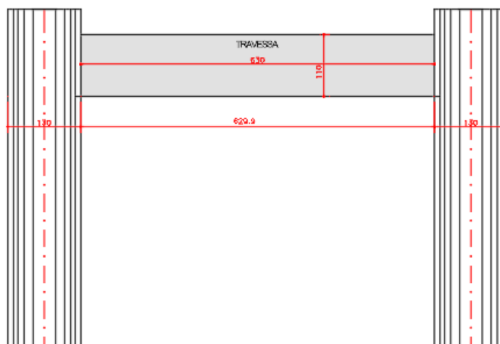
Figura 29 – Detalhe travessas – Proposta 2
