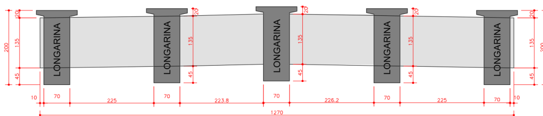
Figura 13 – Detalhe das transversinas apoio – Proposta 1
