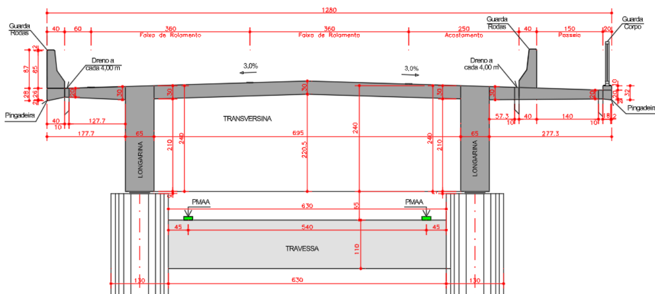
Figura 20 – Corte transversal da estrutura – Proposta 2
