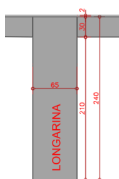
Figura 22 – Detalhe das longarinas – Proposta 2
