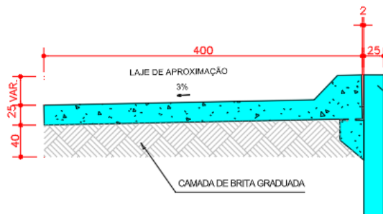
Figura 18 – Detalhe das lajes de aproximação – Proposta 1
