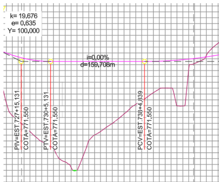
Figura 7 – Situação em Perfil
