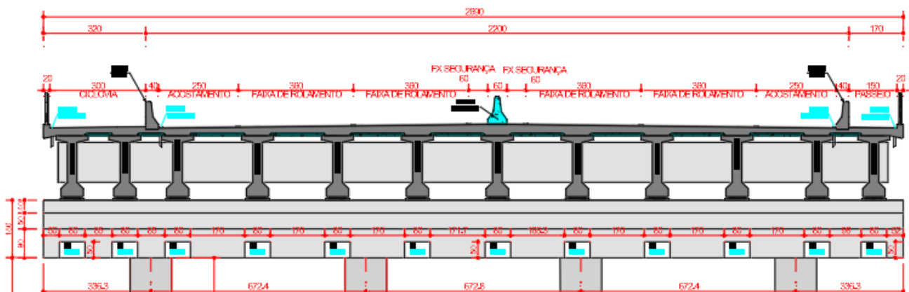
Figura 10 - Corte transversal da estrutura – Proposta 1
