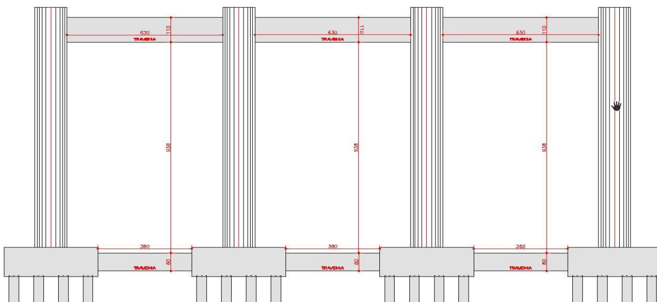
Figura 29 – Detalhe travessas – Proposta 2
