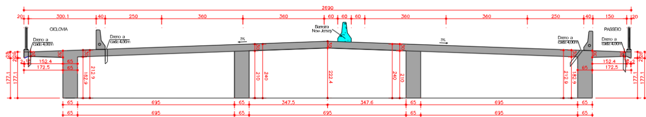
Figura 27 – Detalhe lajes – Proposta 2
