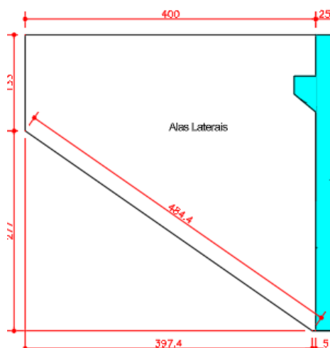
Figura 17 – Detalhe alas – Proposta 1
