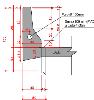
Figura 28 – Drenos e pingadeira – Proposta 1
