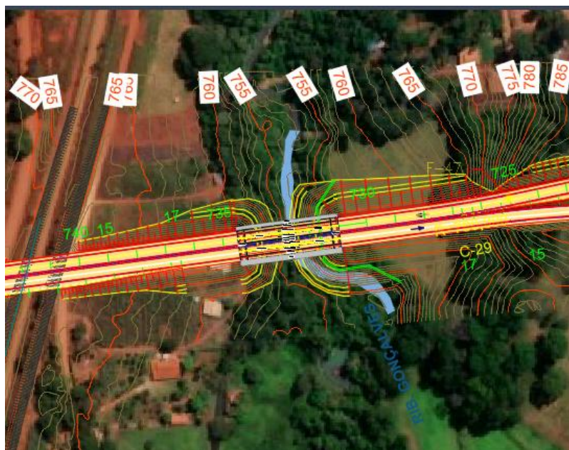
Figura 5 - Planta de localização
