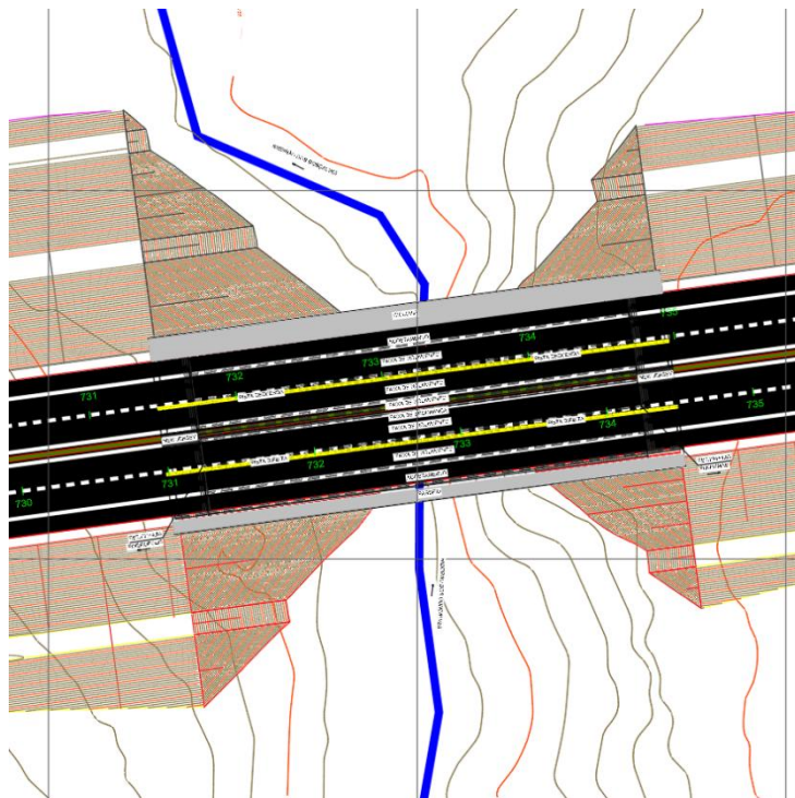
Figura 3 – Planta de Localização da OAE Projetada
