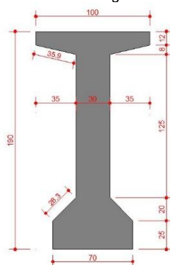
Figura 12 - Detalhes das longarinas – Proposta 1
