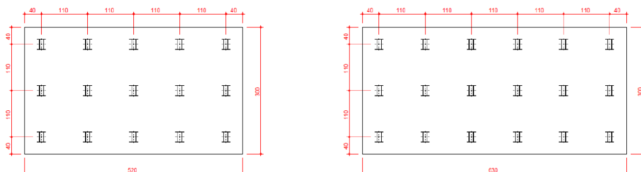
Figura 31 – Detalhe dos blocos de fundação – fundação proposta 2
