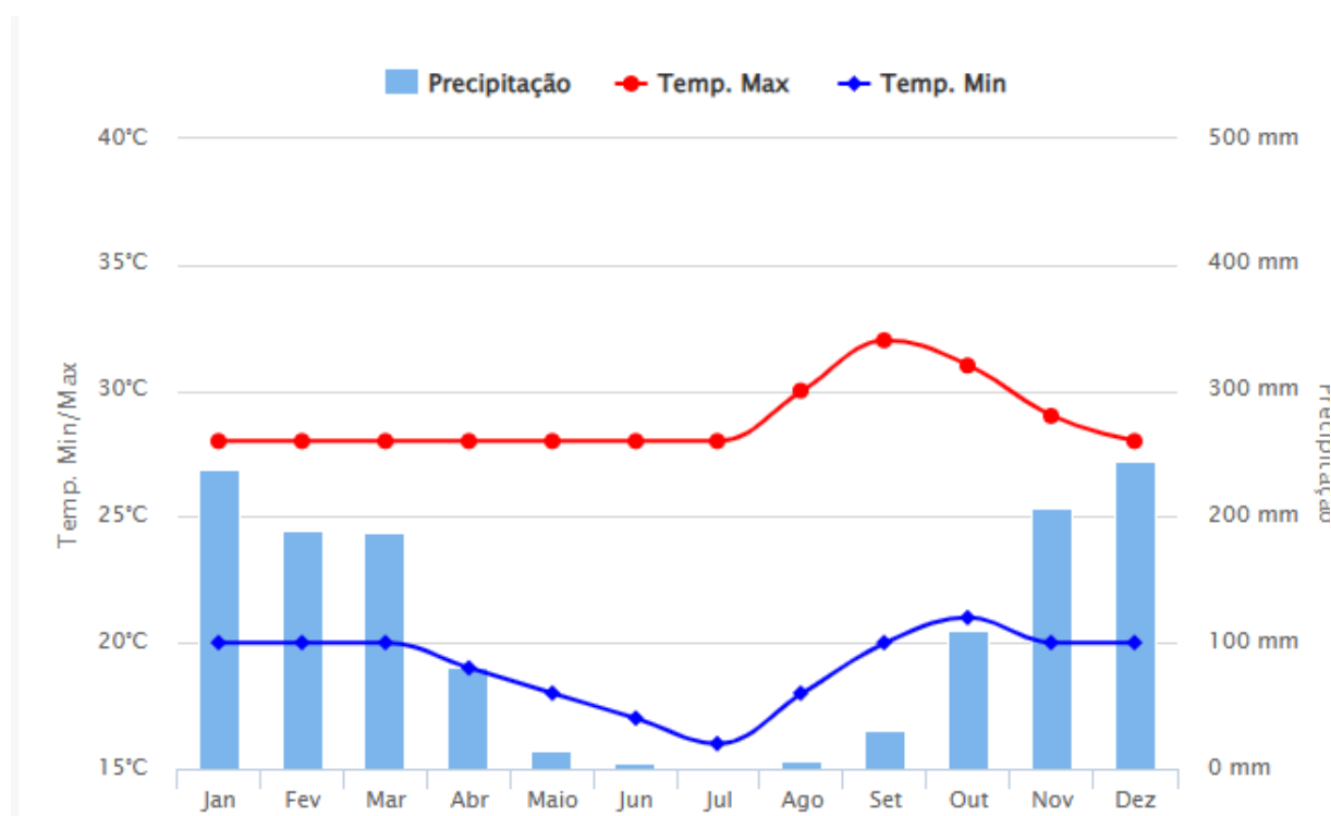
Figura 24 — Gráfico com a série mensal de precipitação (colunas) e temperaturas mín./máx. (linhas)
