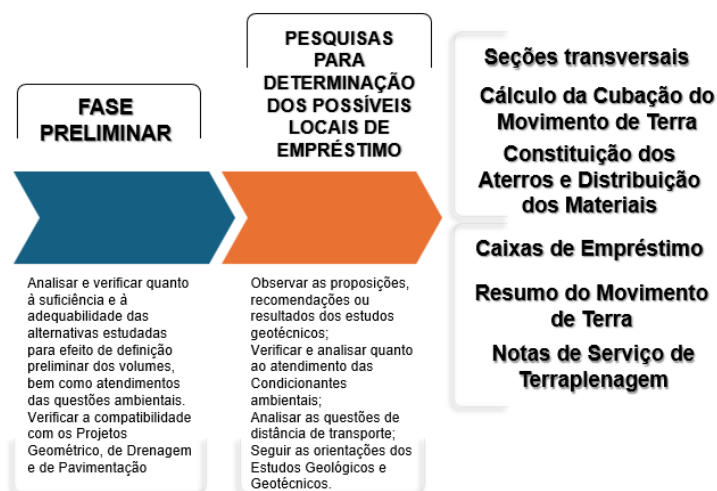
Figura 38 — Roteiro para elaboração do Projeto de Terraplenagem
