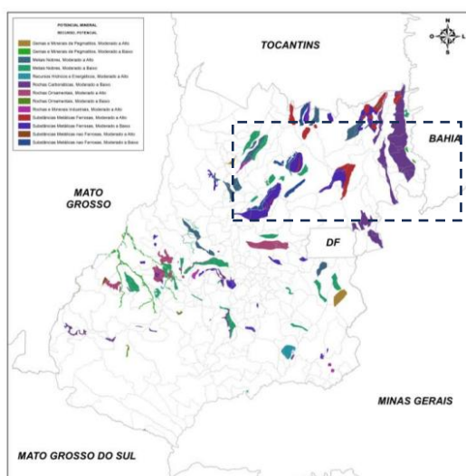
Figura 9 — Mapa com a caracterização mineral do Estado de Goiás com destaque da região de interesse
