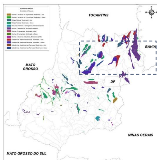
Figura 16 — Mapa com a caracterização mineral do Estado de Goiás com destaque da região de interesse
