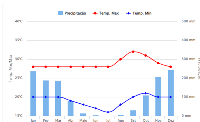
Figura 6 — Gráfico com a série mensal de precipitação (colunas) e temperaturas mín./máx. (linhas)
