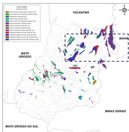
Figura 20 — Mapa com a caracterização mineral do Estado de Goiás com destaque da região de interesse
