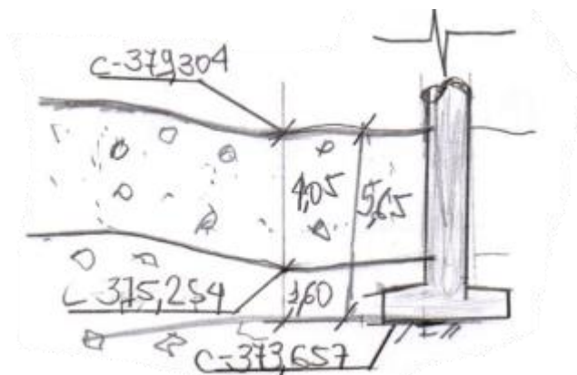
PERFIL
