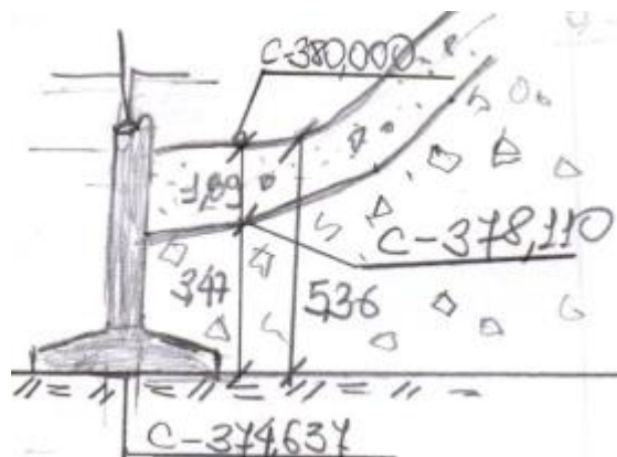
PERFIL
