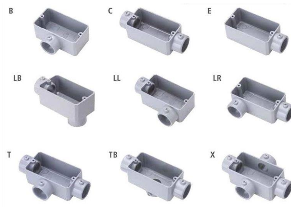
Figura 9 - Tipos de condutor (Ref. Tramontina, Elenco, DAISA)
