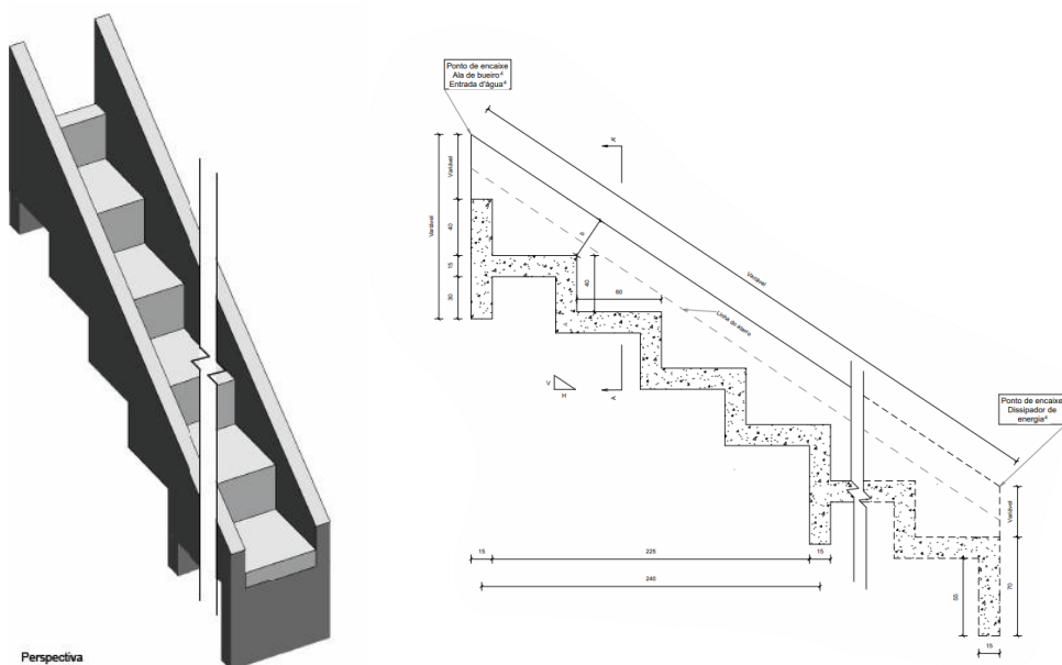
Figura 50: Descida d'água de aterros em degraus – (DAD 60-36)
