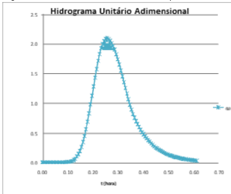
Figura 27 - Gráfico HUT (Autor)
