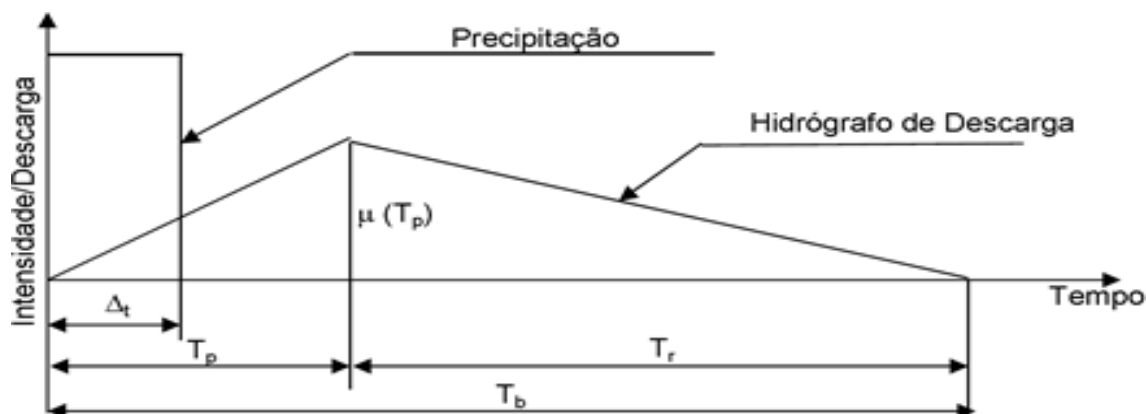
Figura 28 – Principais variáveis do Hidrograma Triangular (Autor).
