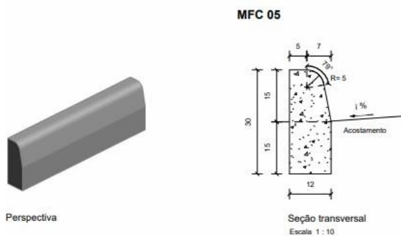
Figura 41: Meio fio com sarjeta - MFC-05
