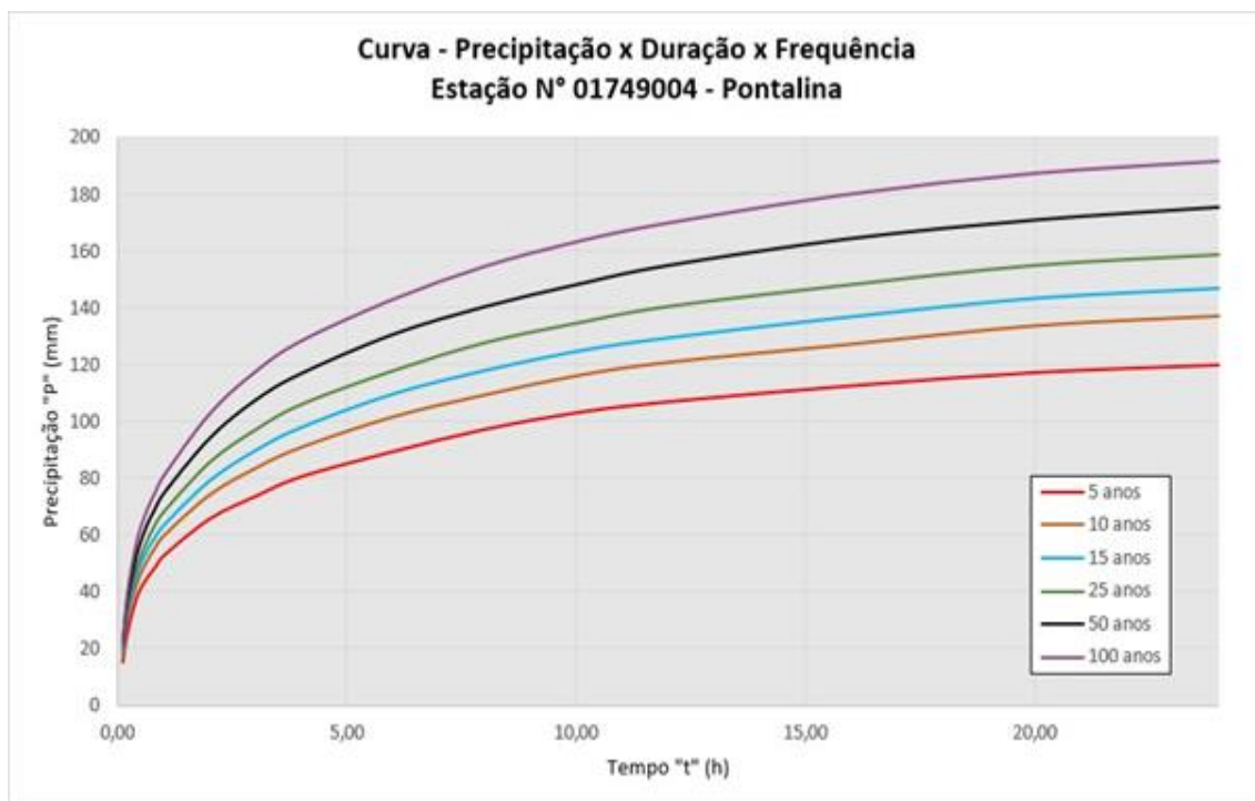
Figura 25 - Precipitação x Duração x Frequência.
