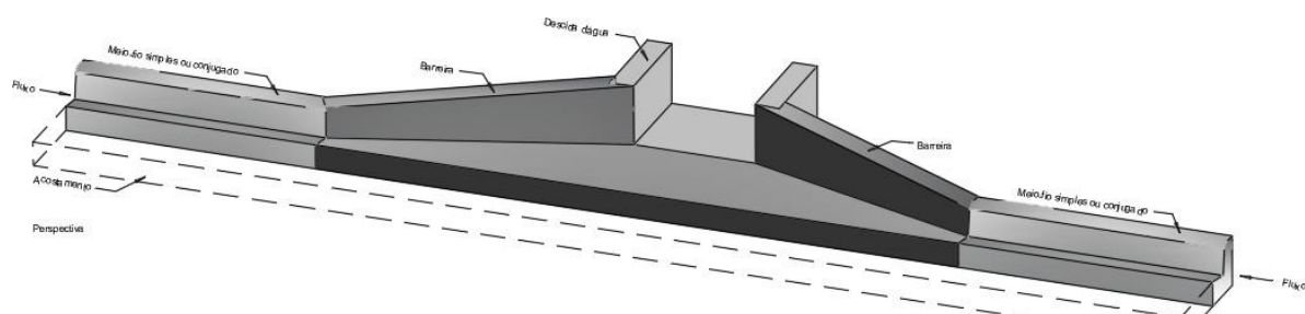
Figura 48: Entradas d'água – Ponto Baixo
