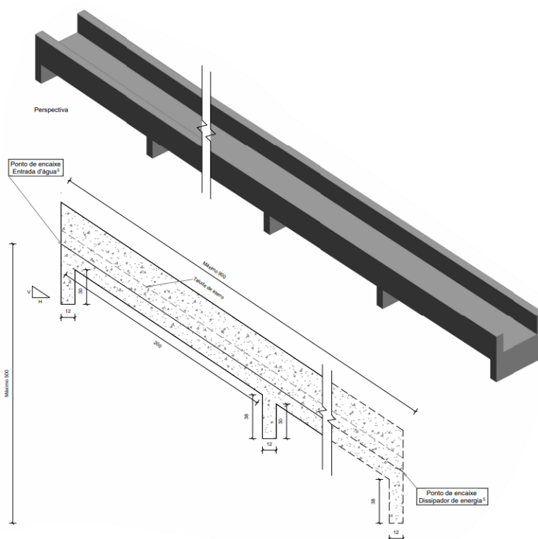
Figura 49: Descida d'água de aterros tipo rápido (lisa) – (DAR 60-30)
