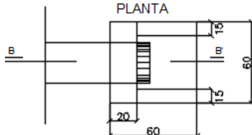
Figura 52: Bocas de saída em concreto – BSD 02.
