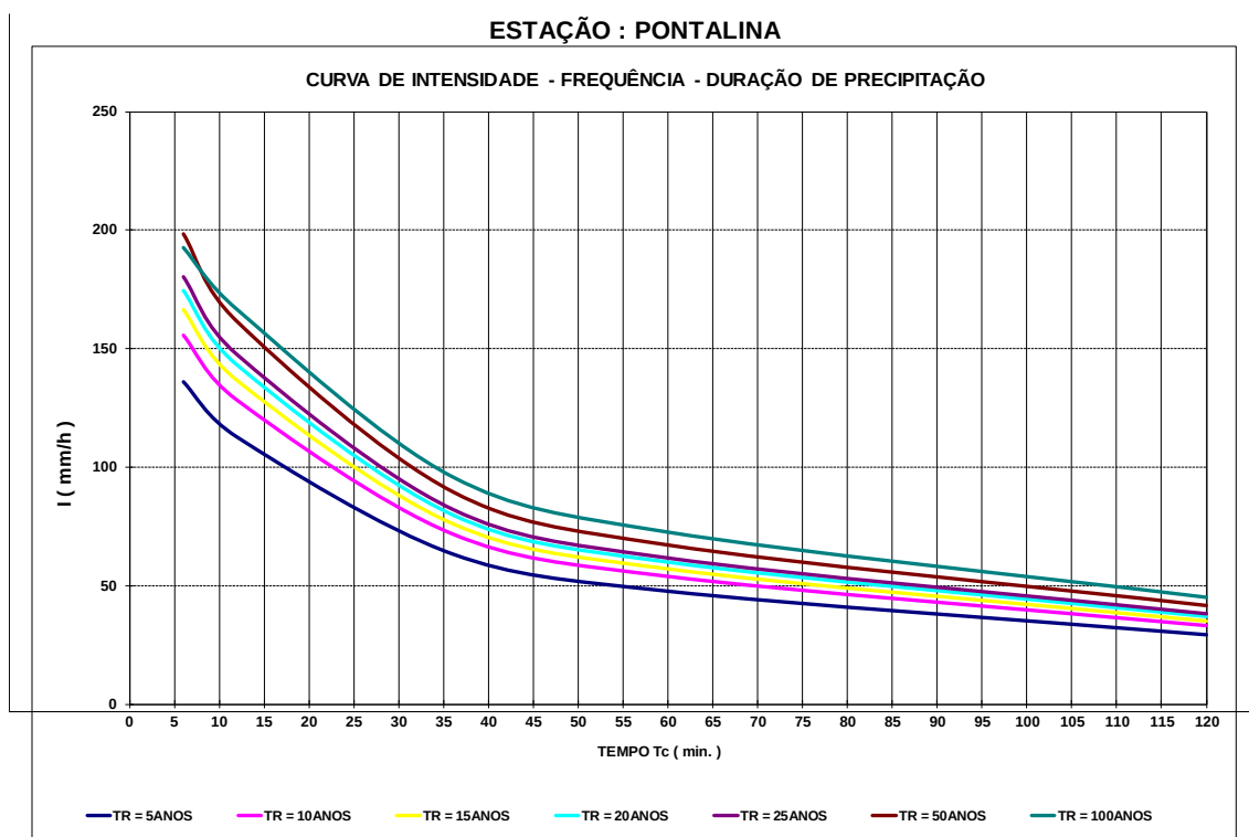
Figura 26 - Intensidade x Duração x Frequência
