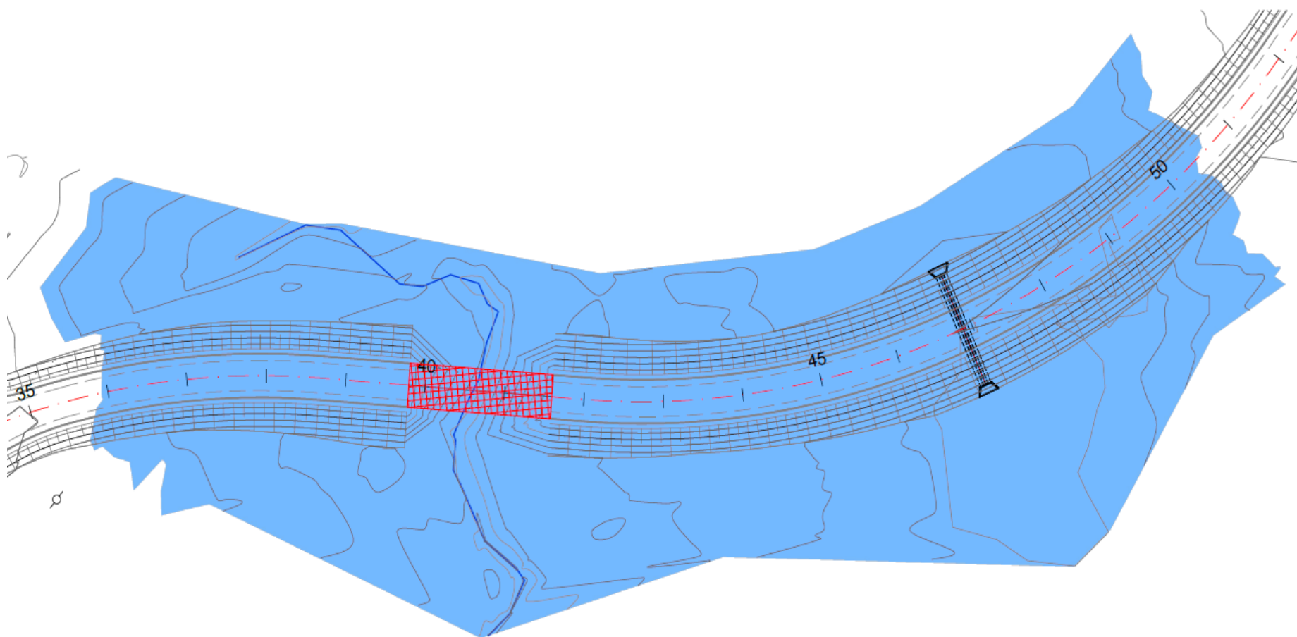
Figura 29 – Mancha de inundação da enchente máxima de projeto
