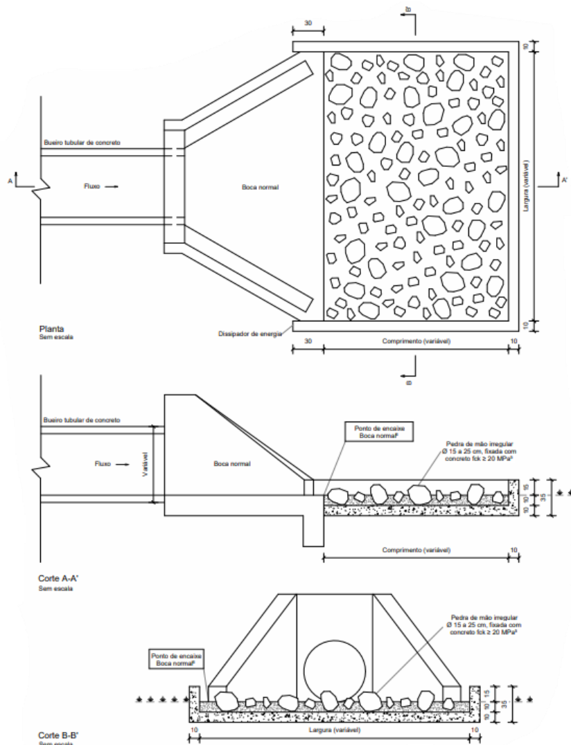
Figura 53: Dissipadores de Energia – DEB
