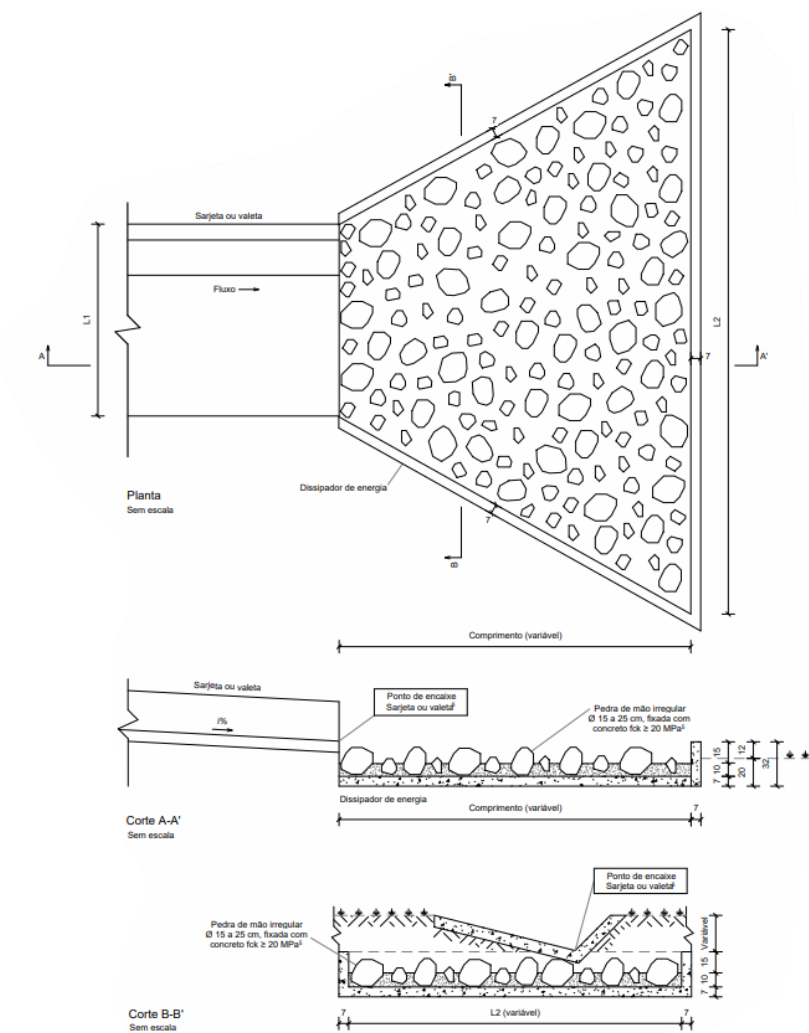
Figura 54: Dissipadores de Energia – DES
