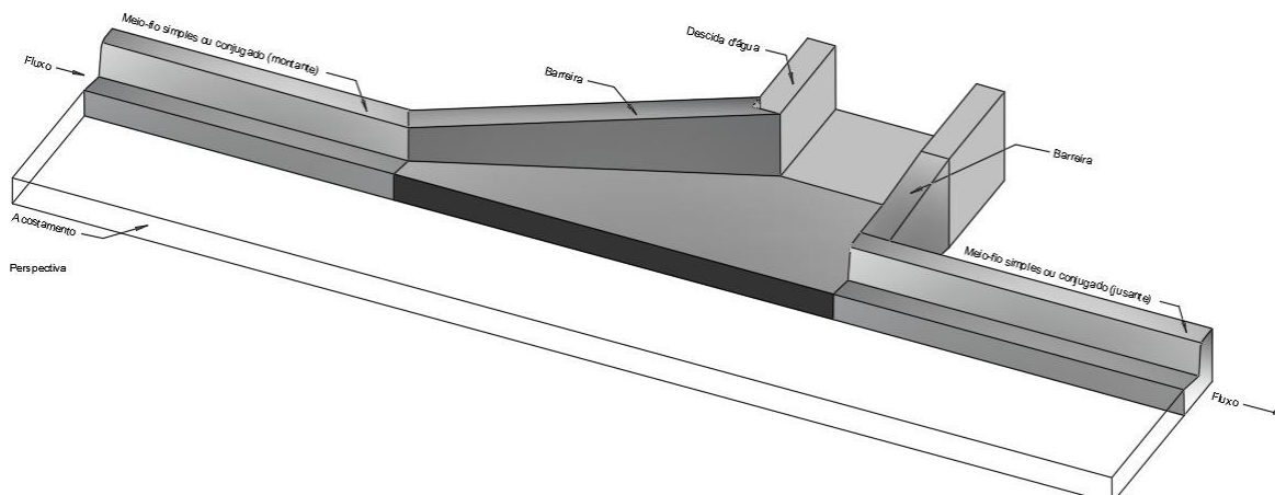
Figura 47: Entradas d'água – Greide Continuo
