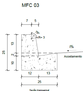
Figura 40: Meio fio com sarjeta - MFC-03
