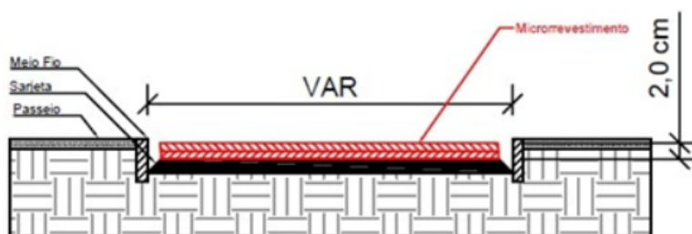
Figura 04 – Esquema de perfil transversal para Microrrevestimento.
