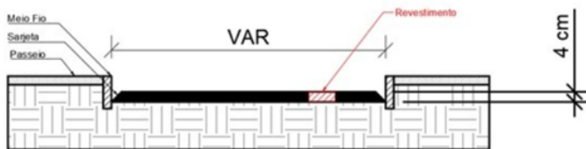
Figura 01 – Esquema de perfil transversal para reparo superficial.
