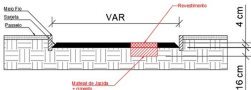
Figura 02 – Esquema de perfil transversal para reparo profundo.
