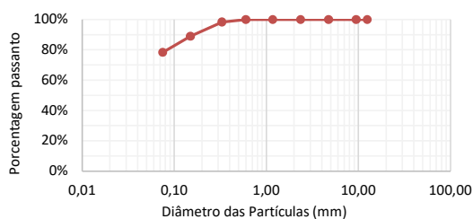
Curva Granulométrica
