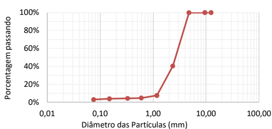
Curva Granulométrica
