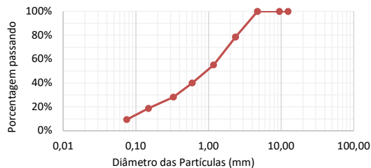
Curva Granulométrica
