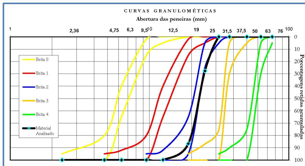
Gráfico das Curvas Granulométricas
