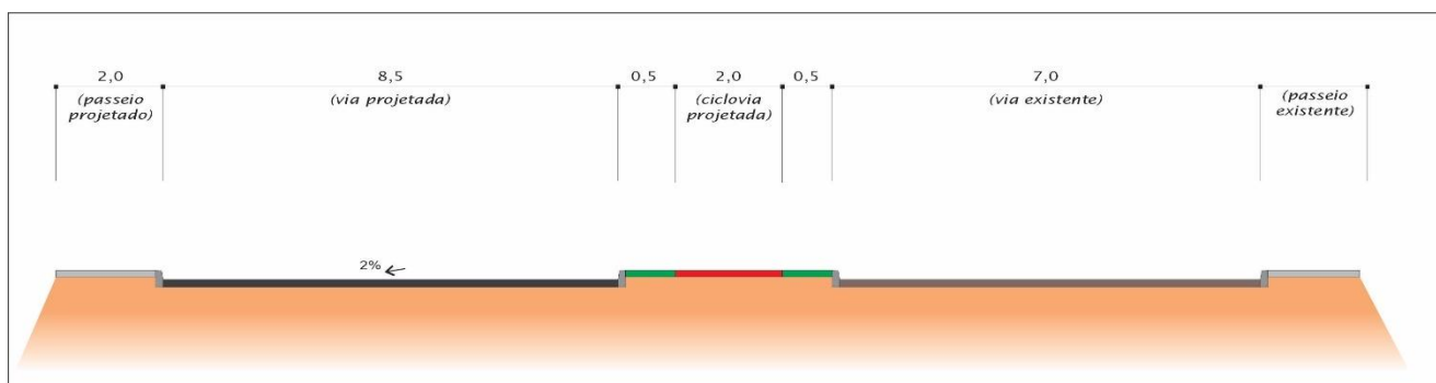
Figura 10: Seção transversal após ribeirão Santo Antônio
