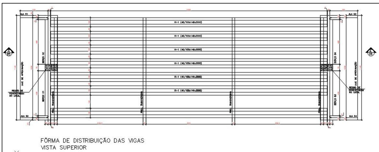
Figura 75: Vista Superior de cada OAE (Fôrma do Tabuleiro).
