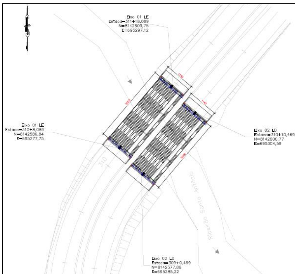
Figura 73: Vista Superior das OAEs projetadas.
