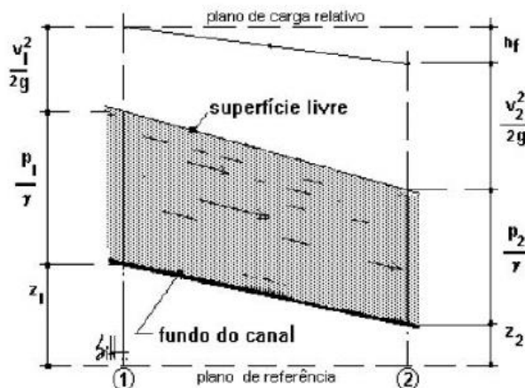
Figura 42 - Escoamento livre (Fonte: FERNANDES, Carlos. 1997).
