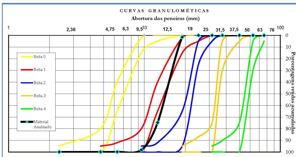
Gráfico das Curvas Granulométricas
