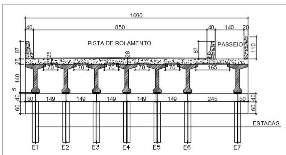
Figura 76: Corte Transversal de cada OAE.
