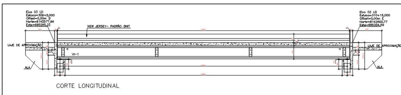
Figura 74: Vista Lateral de cada OAE (Seção Longitudinal).
