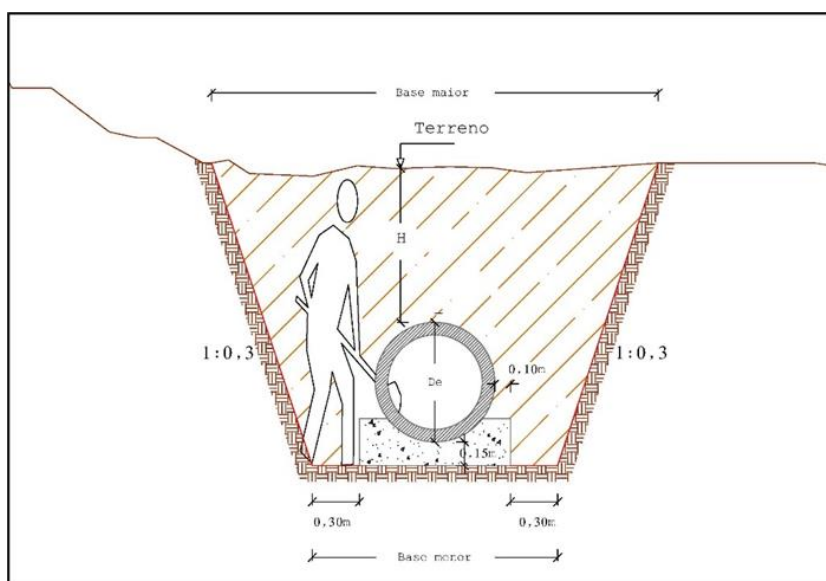
Figura 77 - Representação da escavação em bueiros tubulares.
