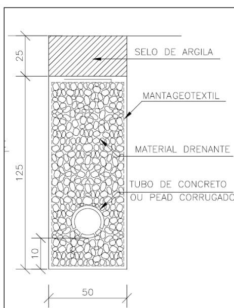
Figura 70 - Dreno DPS07
