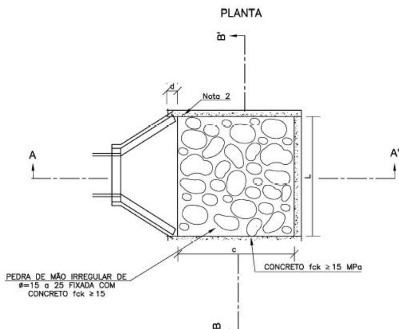
Figura 67 - Dissipadores de energia - DEB01 a DEB13
