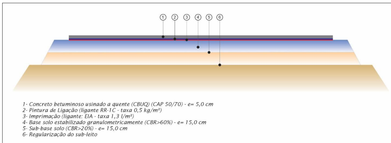
Figura 54: Estrutura de pavimentação
