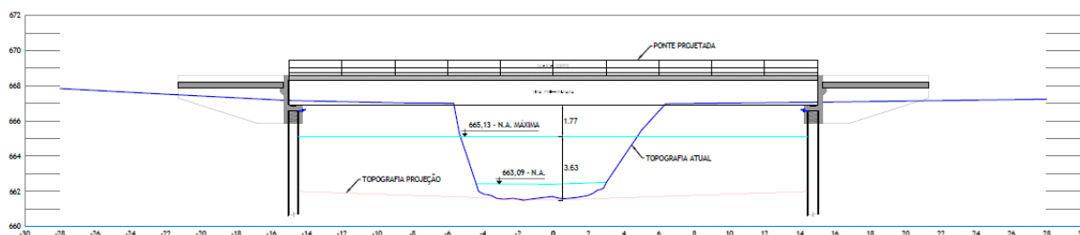
Figura 4443 - Seção transversal ponte sobre o ribeirão Santo Antônio.
