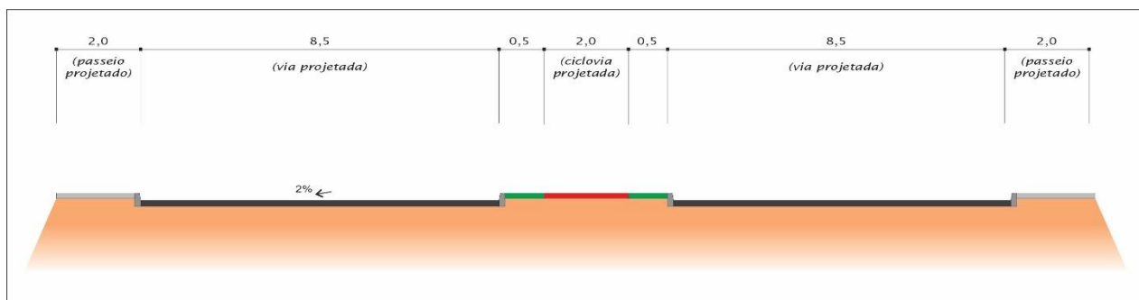
Figura 9: Seção transversal trecho rural
