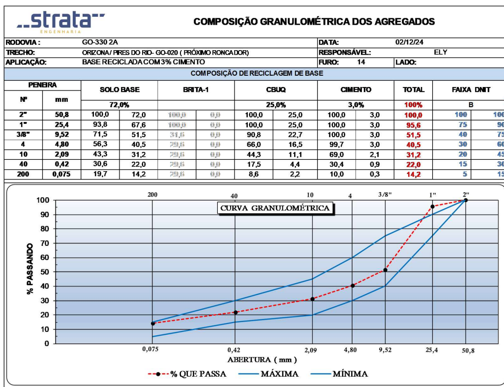
Figura 85 - Gráfico de Composição Granulométrica dos Agregados (Furo 14).
