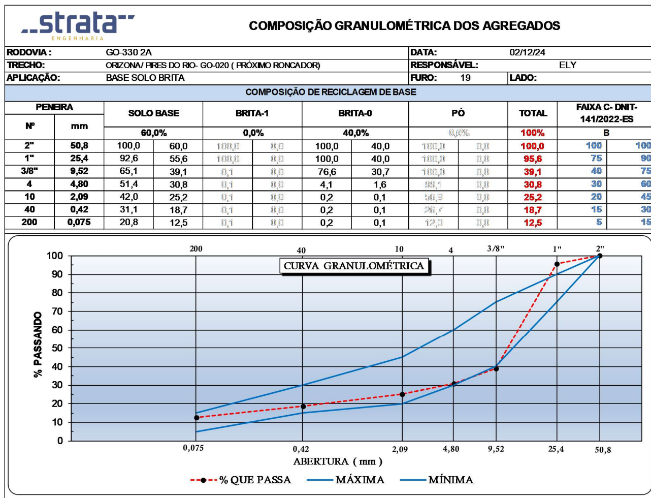
Figura 75 - Gráfico de Composição Granulométrica (Furo 19).
