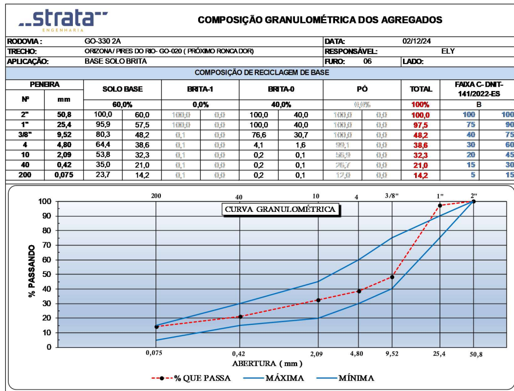
Figura 72 - Gráfico de Composição Granulométrica (Furo 06).
