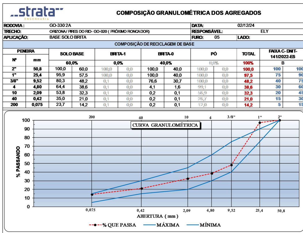
Figura 71 - Gráfico de Composição Granulométrica (Furo 05).
