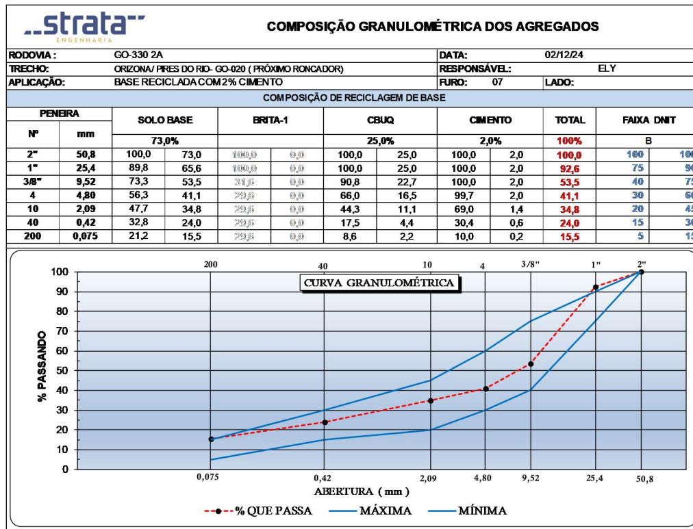
Figura 78 - Gráfico de Composição Granulométrica dos Agregados (Furo 07).
