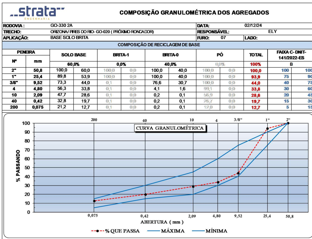
Figura 73 - Gráfico de Composição Granulométrica (Furo 07).
