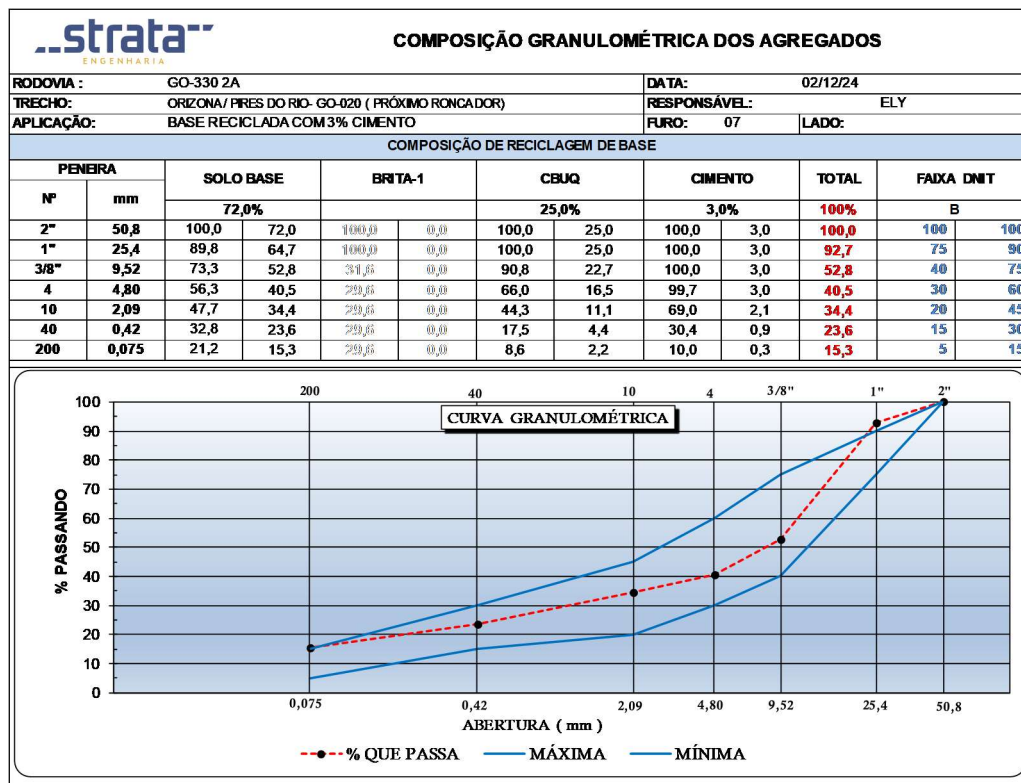
Figura 84 - Gráfico de Composição Granulométrica dos Agregados (Furo 07).
