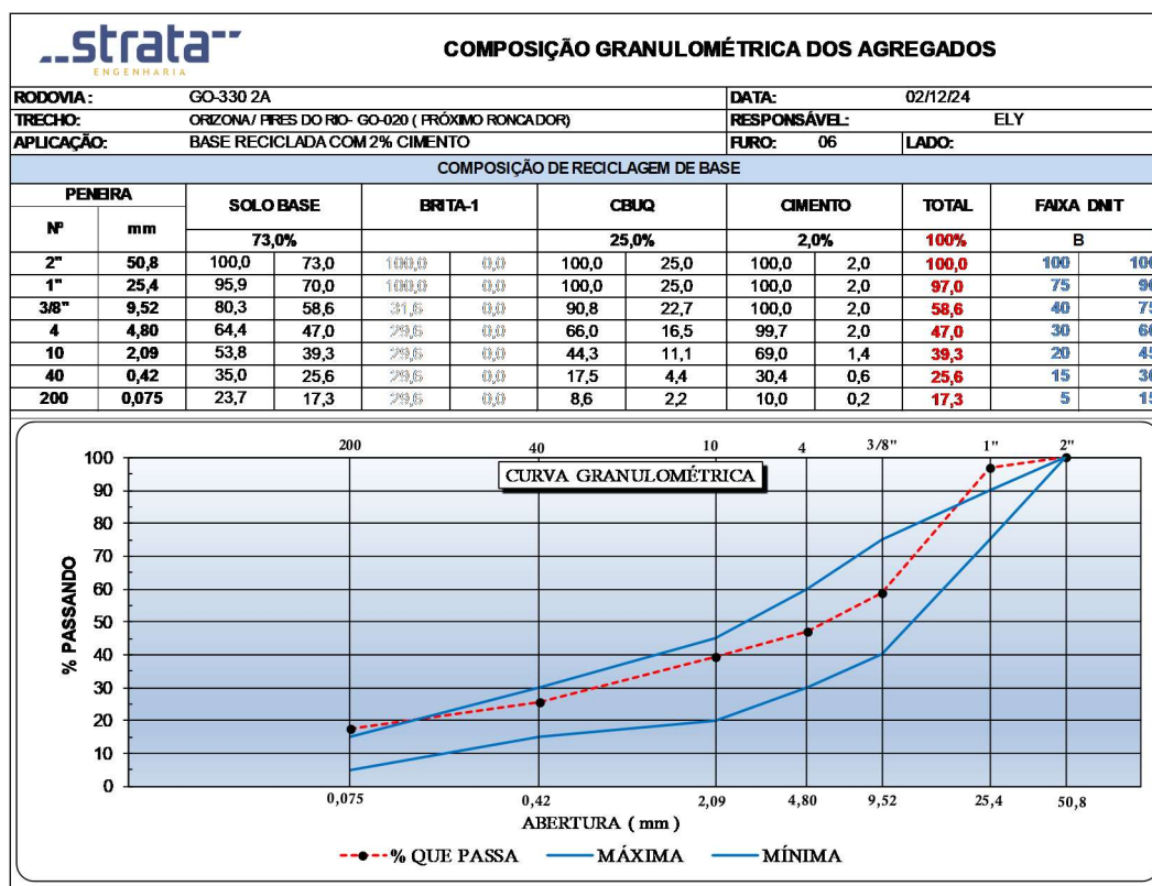
Figura 77 - Gráfico de Composição Granulométrica dos Agregados (Furo 06).
