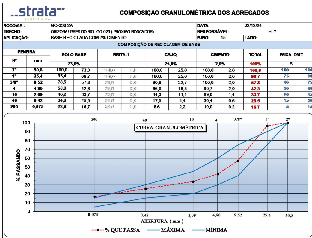
Figura 80 - Gráfico de Composição Granulométrica dos Agregados (Furo 15).
