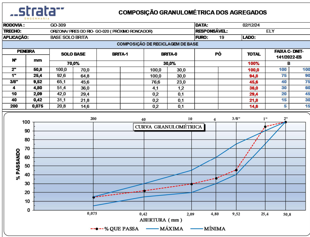
Figura 69 - Gráfico de Composição Granulométrica (Furo 19).
