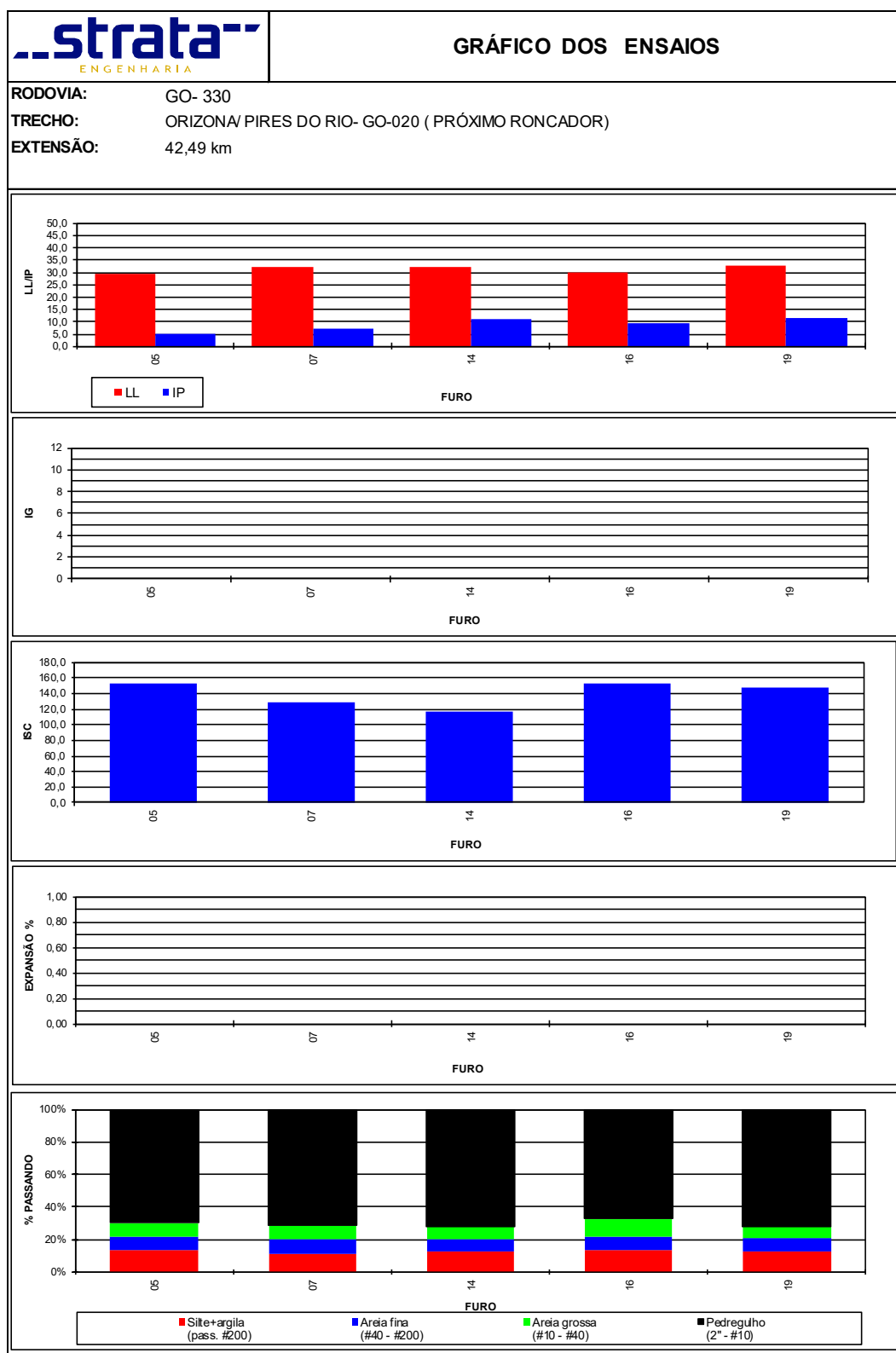
Figura 64 - Gráfico dos Ensaio (Base + 30% de Brita).
