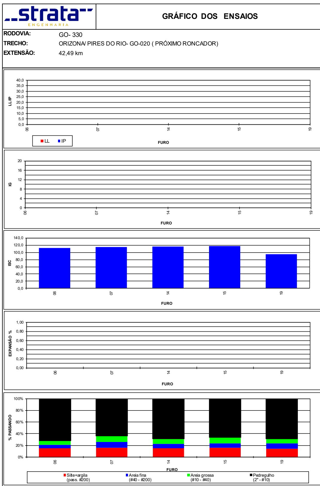
Figura 76 - Gráfico dos Ensaiois (Base com Incorporação de Revestimento + 2% de Cimento).
