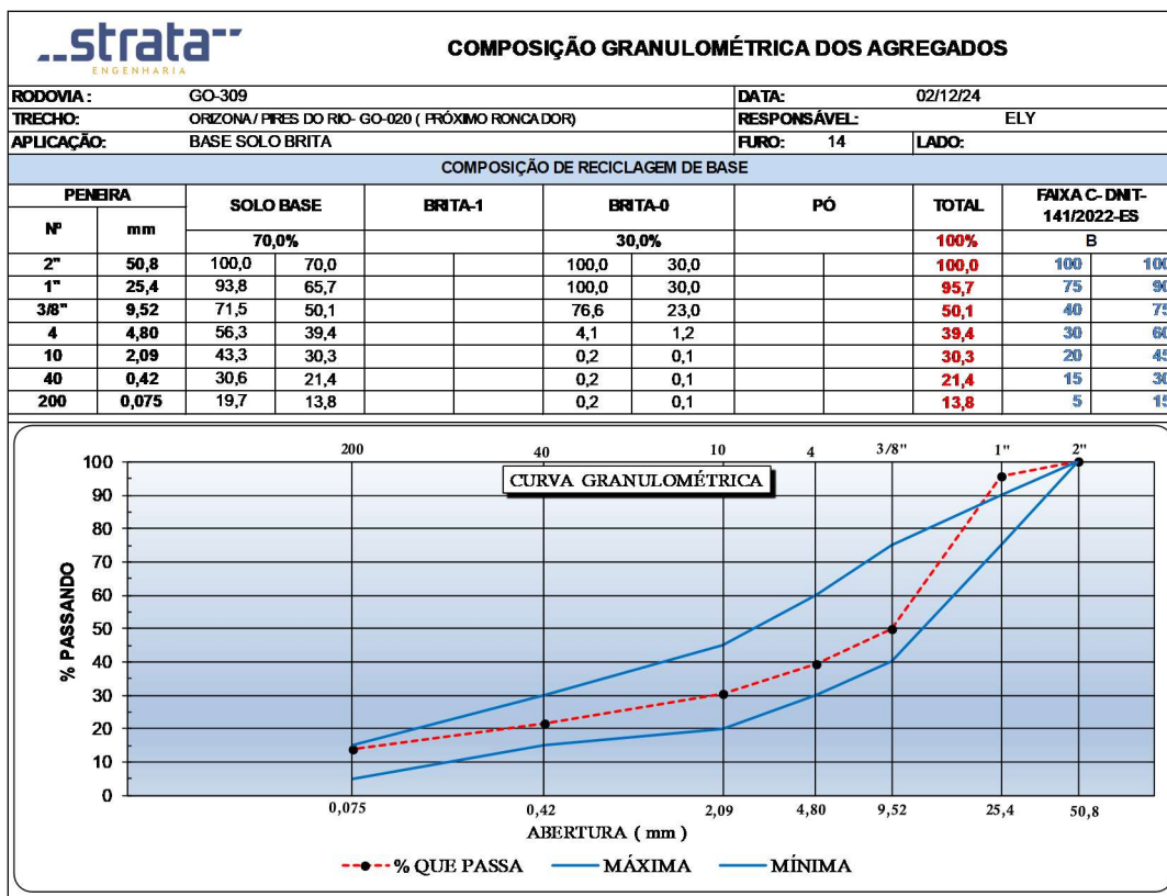
Figura 67 - Gráfico de Composição Granulométrica (Furo 14).
