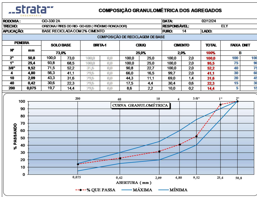
Figura 79 - Gráfico de Composição Granulométrica dos Agregados (Furo 14).
