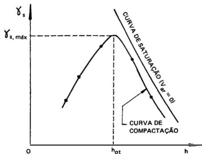
Figura 21 - Curva de Compactação.
