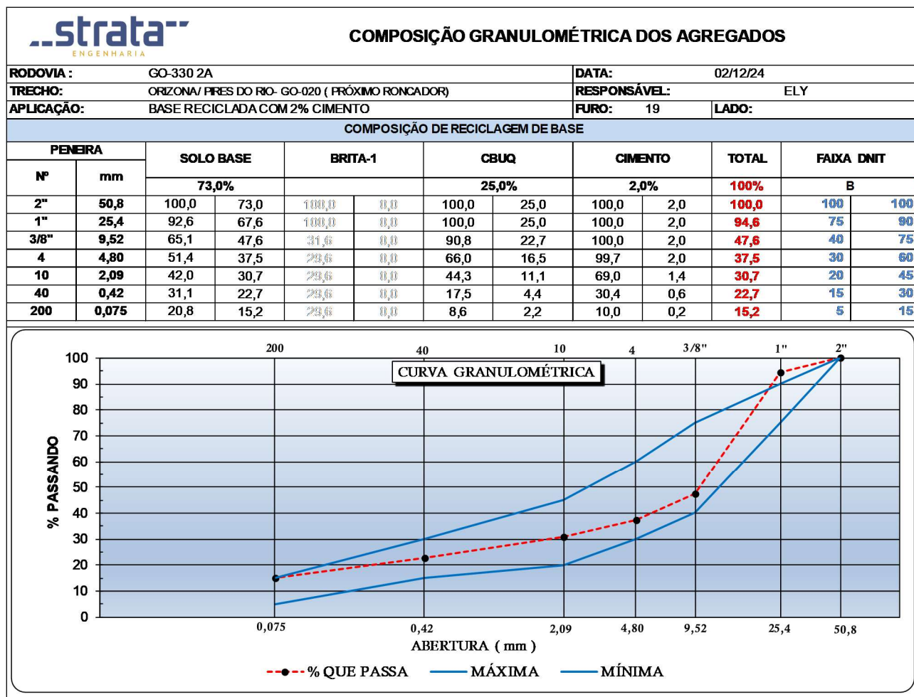
Figura 81 - Gráfico de Composição Granulométrica dos Agregados (Furo 19).
