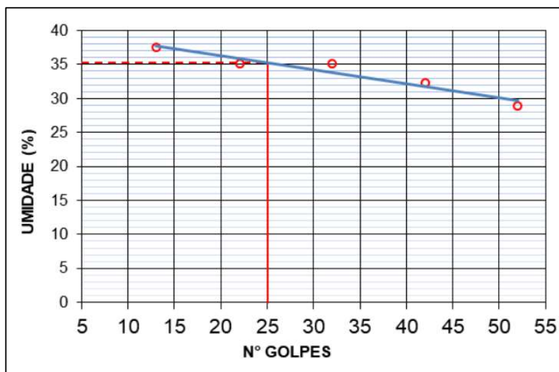
Figura 18 - Gráfico do Limite de Liquidez.
