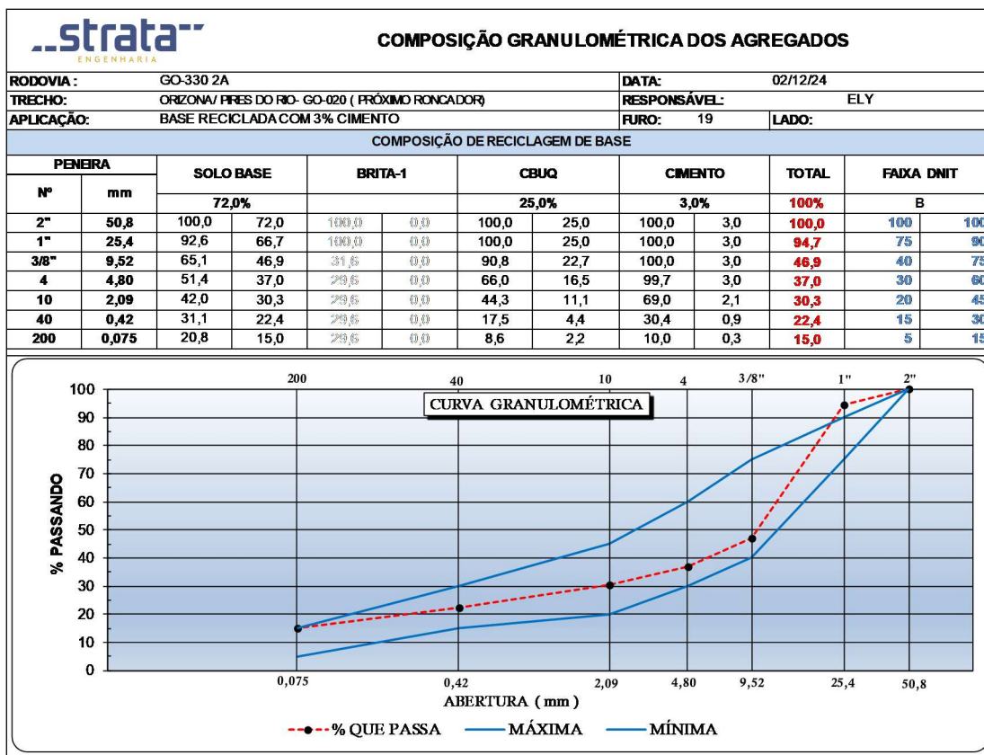
Figura 87 - Gráfico de Composição Granulométrica dos Agregados (Furo 19).
