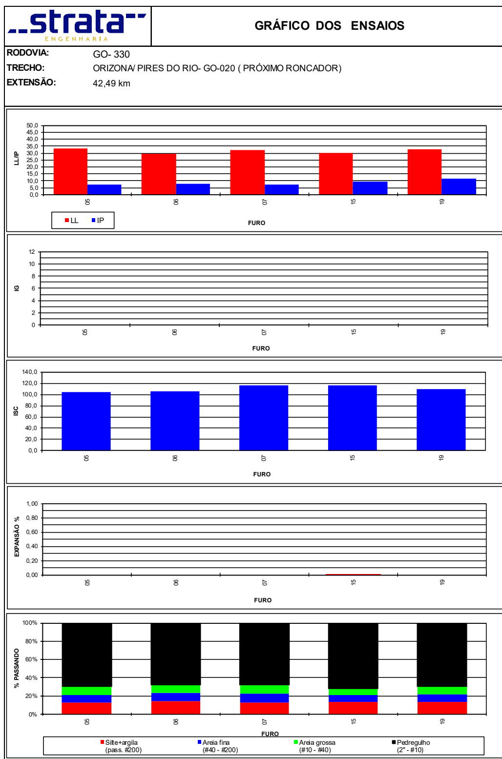
Figura 70 - Gráfico dos Ensaios (Base + 40% de Brita).
