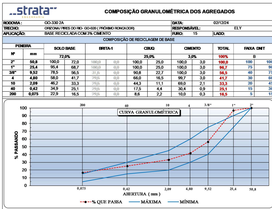
Figura 86 - Gráfico de Composição Granulométrica dos Agregados (Furo 15).
