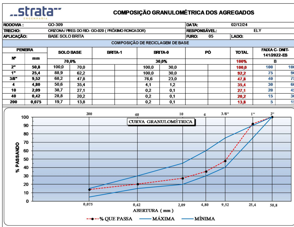
Figura 65 - Gráfico de Composição Granulométrica (Furo 05).
