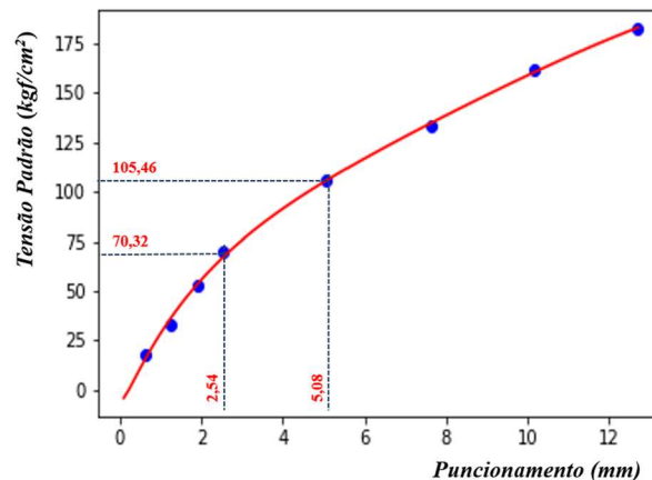
Figura 25 - Curvas CBR (carga x punção).
