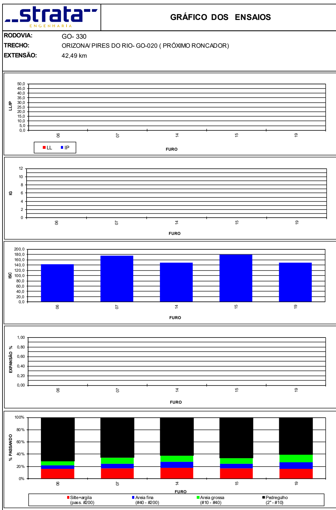
Figura 82 - Gráfico dos Ensaio (Base com Incorporação de Revestimento + 3% de Cimento).
