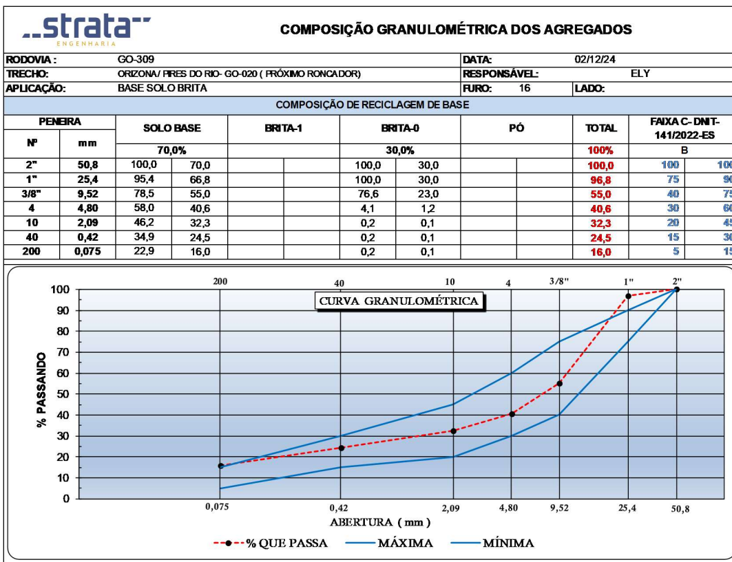
Figura 68 - Gráfico de Composição Granulométrica (Furo 16).
