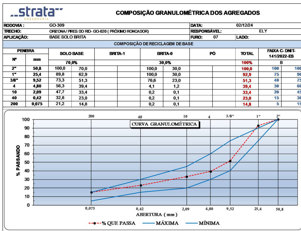
Figura 66 - Gráfico de Composição Granulométrica (Furo 07).
