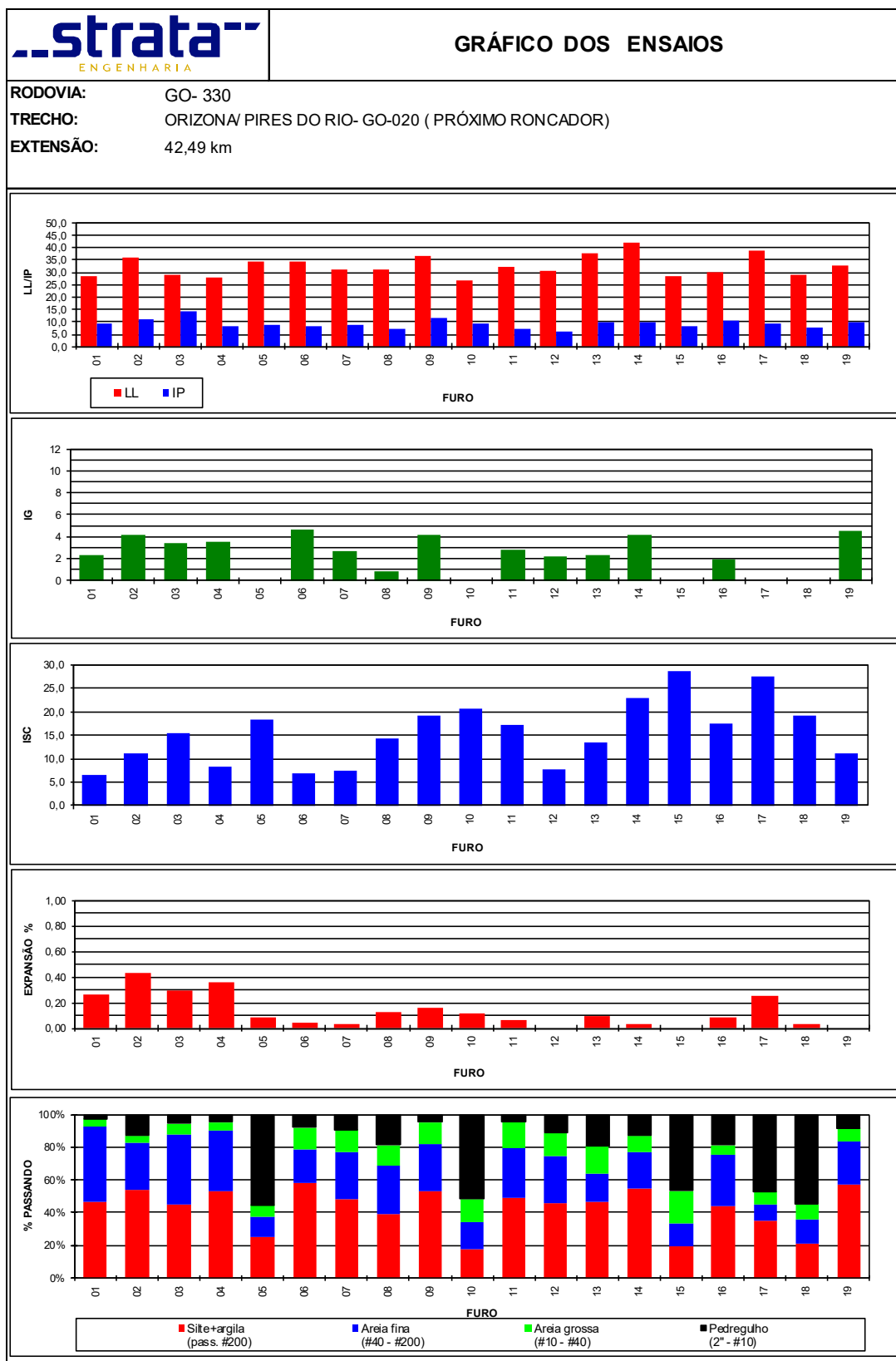
Figura 29 - Gráfico dos Ensaios Subleito.
