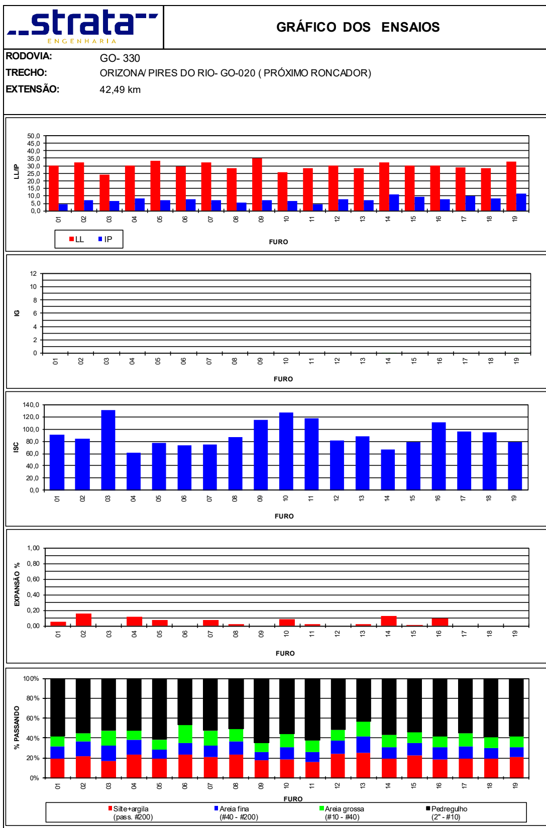
Figura 27 - Gráfico dos Ensaios Base.
