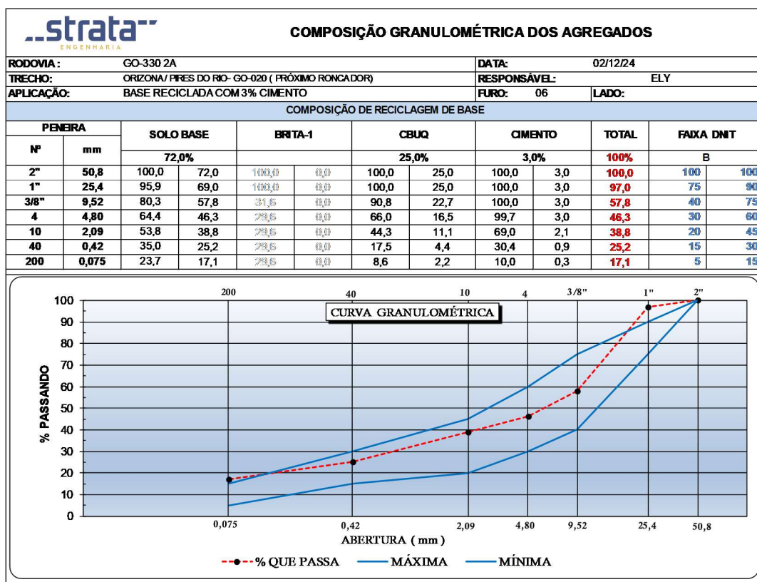
Figura 83 - Gráfico de Composição Granulométrica dos Agregados (Furo 06).
