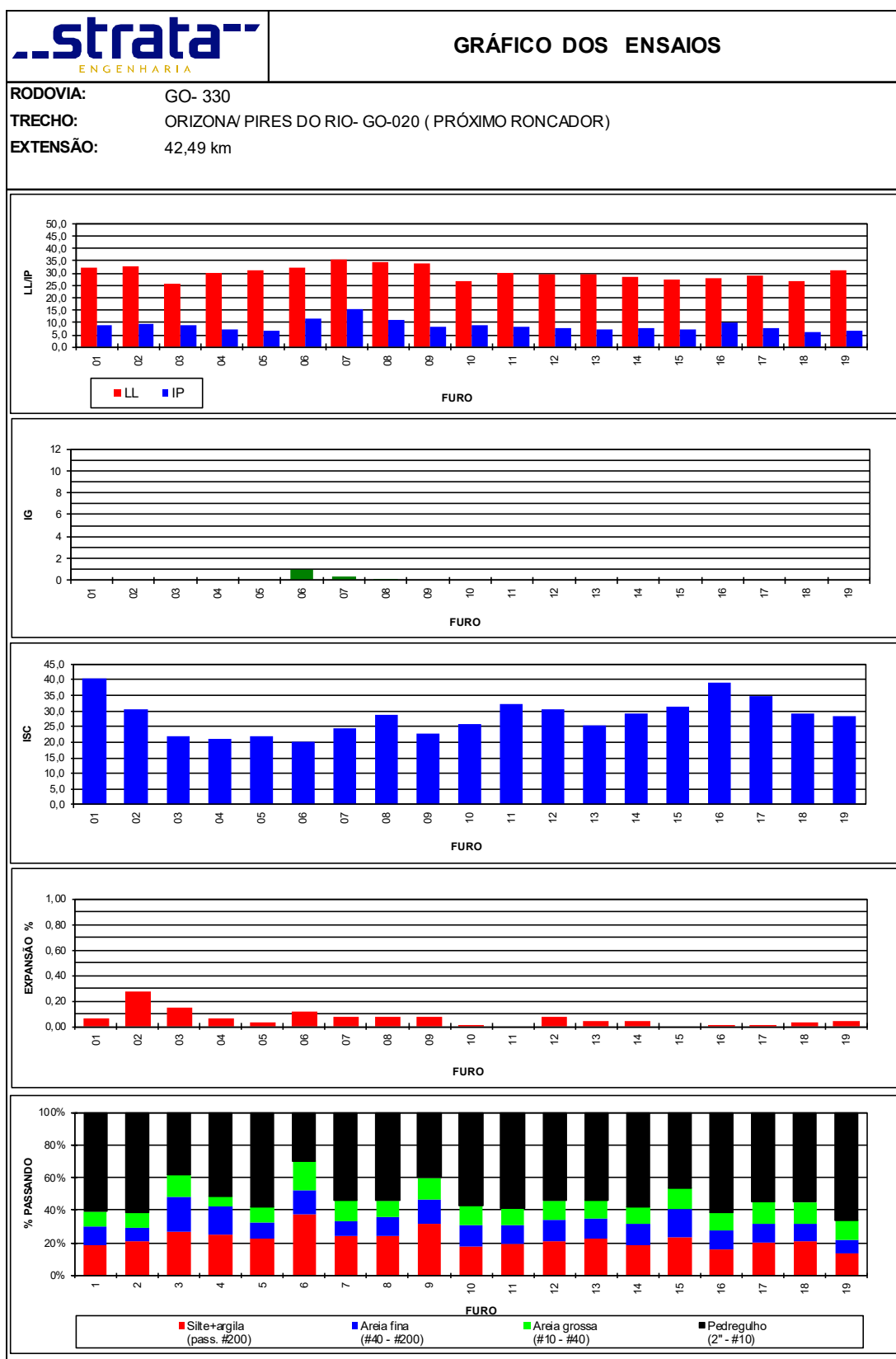
Figura 28 - Gráfico dos Ensaios Sub-base.
