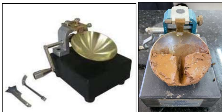
Figura 16 - Aparelho de Casagrande.
