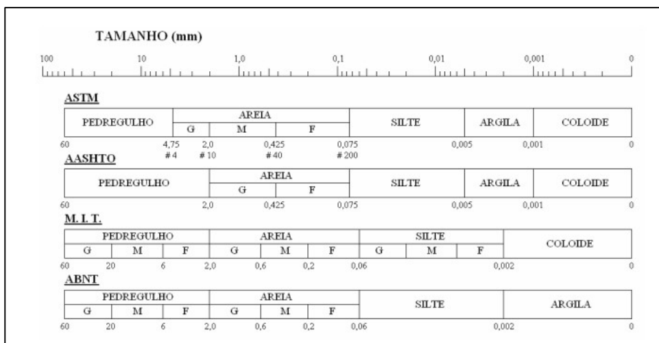
Figura 13- Distinção do Tamanho dos Materiais
