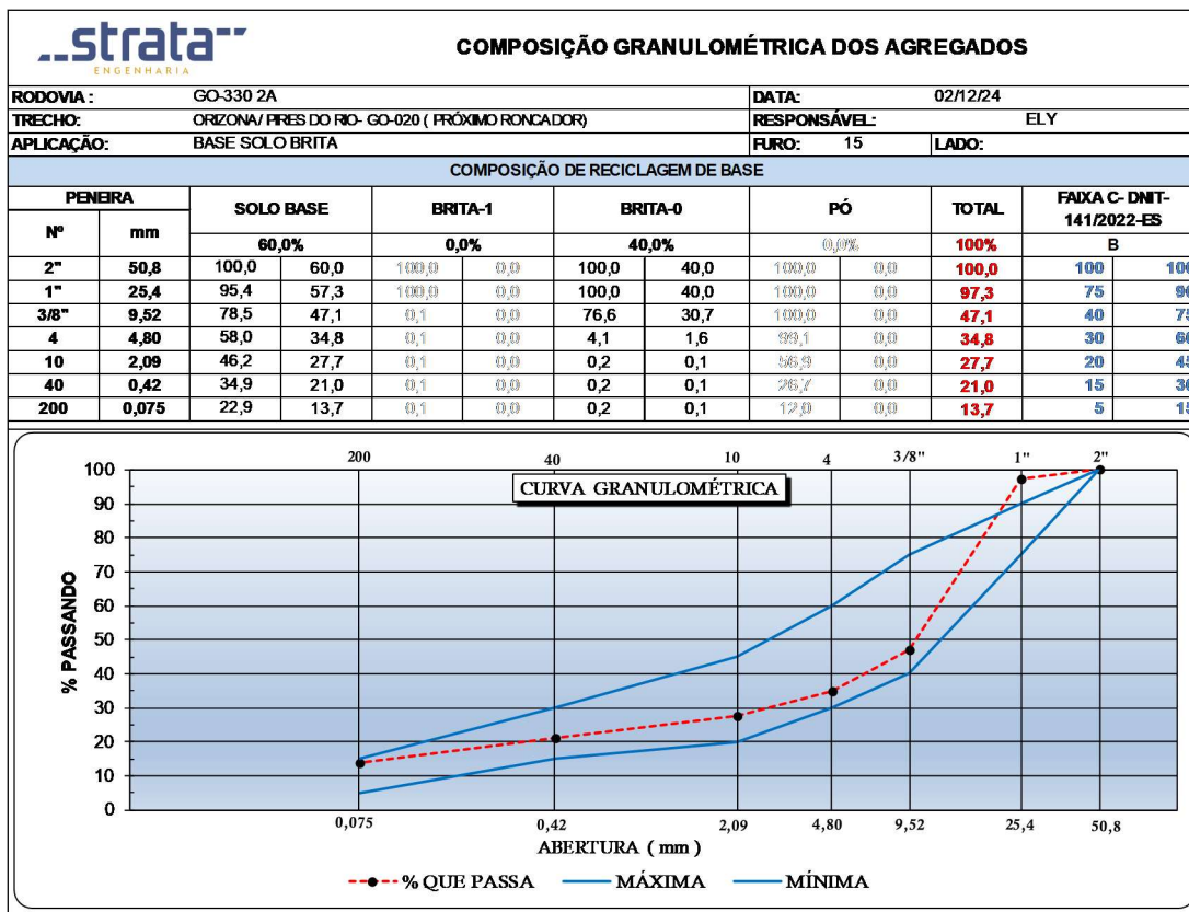
Figura 74 - Gráfico de Composição Granulométrica (Furo 15).
