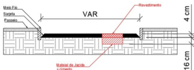
Figura 02 – Esquema de perfil transversal para reparo profundo.
