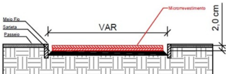
Figura 04 – Esquema de perfil transversal para Microrrevestimento.
