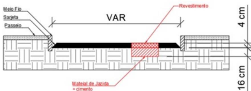
Figura 02 – Esquema de perfil transversal para reparo profundo.
