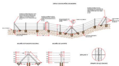
CERCA - 5 FIOS
