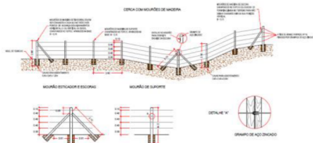
CERCA - 4 FIOS
